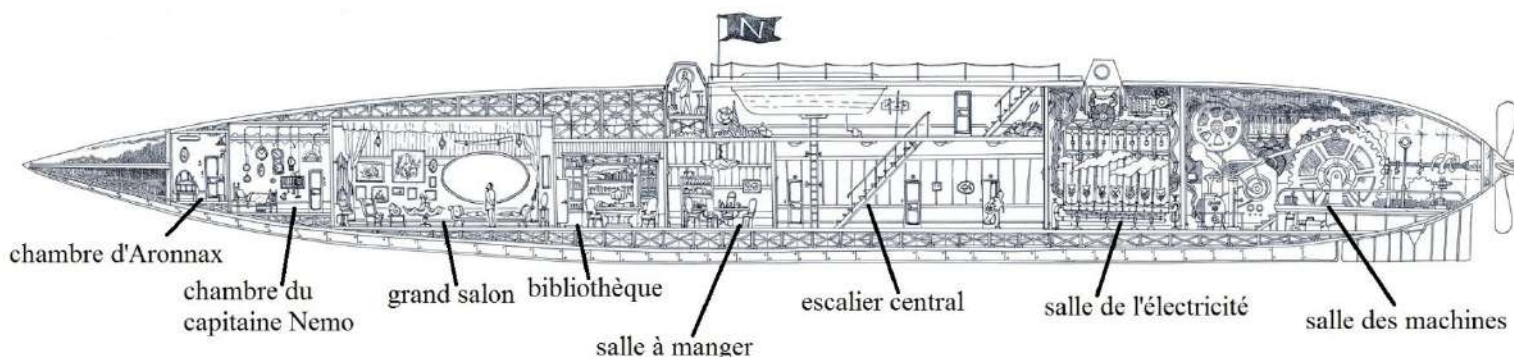
Plan de coupe du Nautilus de Jean-Marc Deschamps, Le Nautilus , Paris, Éditions Vagon du Plaisancier, 2017, pp.20-21.
