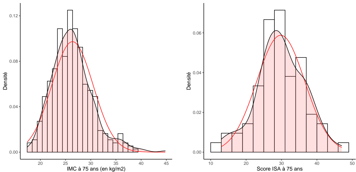
FIGURE 3: Histogramme de la distribution de l'IMC (à gauche, n=371 ) et du IST (à droite, n=70 ) pour les sujets à 75 ans de l'étude 3C dans la sélection de Bordeaux, distribution normale en rouge et distribution observée en rose pâle.
