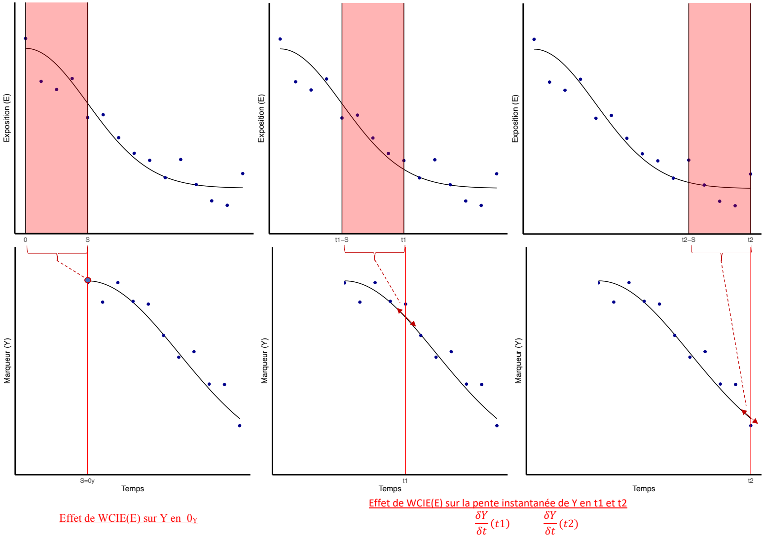
FIGURE 1: Schéma explicatif du modèle conjoint de l'histoire d'une exposition E et d'un marqueur Y pour un sujet.
