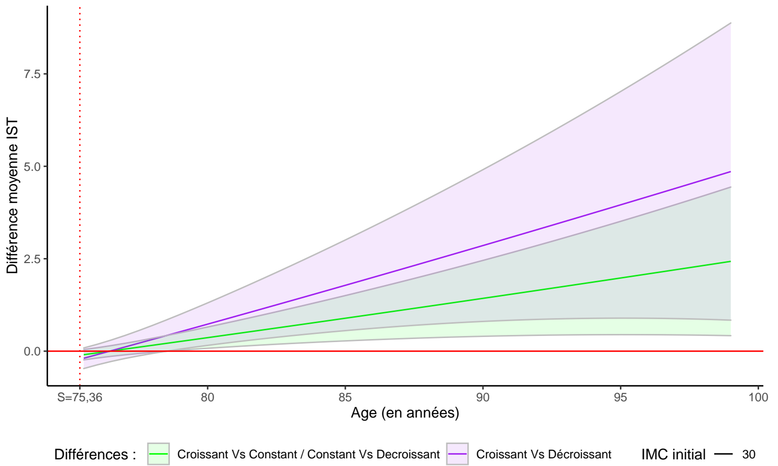
FIGURE 10: Courbes des différences prédites d'IST pour un IMC initial à 30 \text{ kg}/\text{m}^2 avec divers profils d'évolution de l'IMC chez un homme, sans gène APOE4, ayant fait des études courtes et rentrant dans l'étude à 64 ans.
