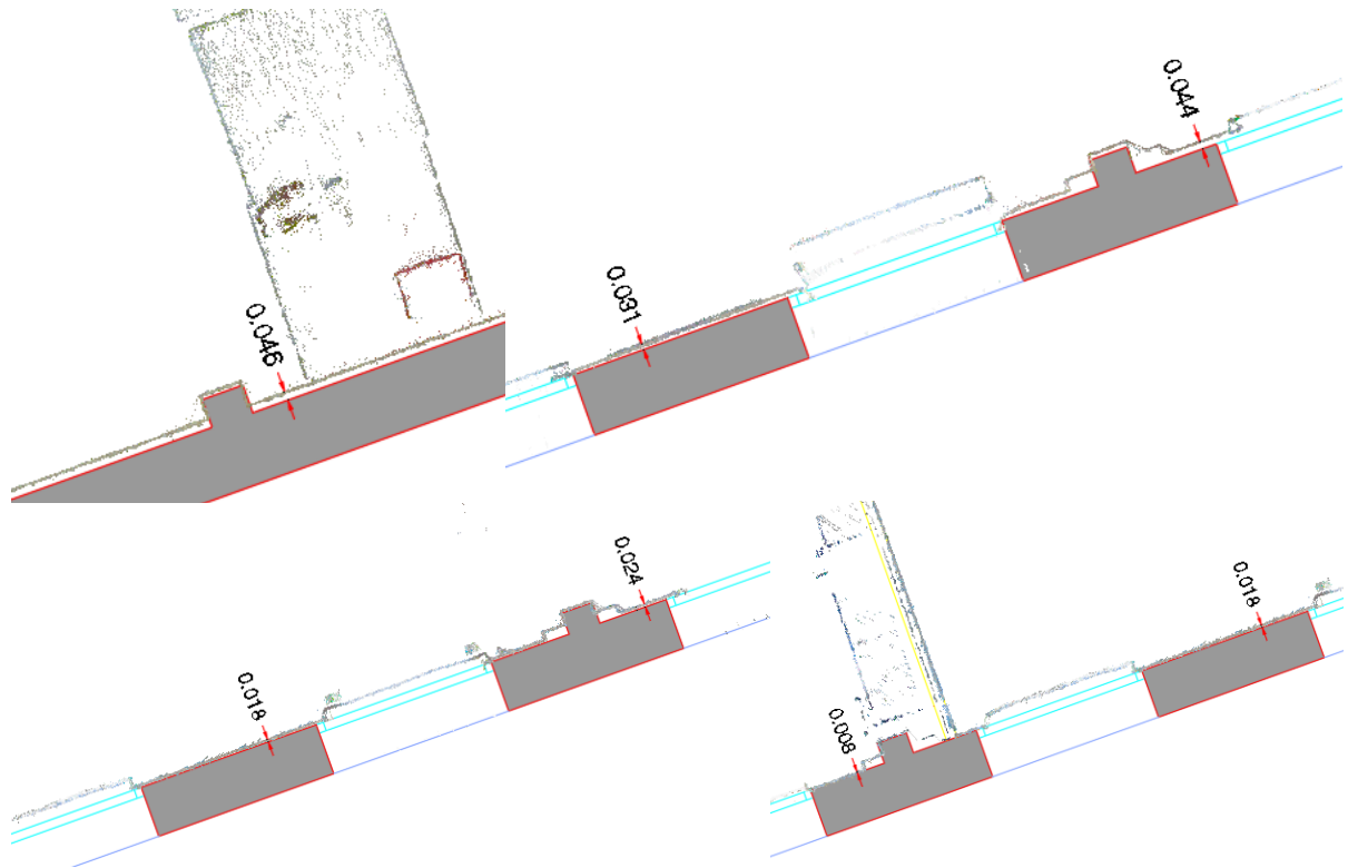
Figure 20 : Capture d'écran du logiciel Autocad, de l'écart entre le nuage de points et le plan au 1/100 ième choisi comme référence. Source N. Amadiou
