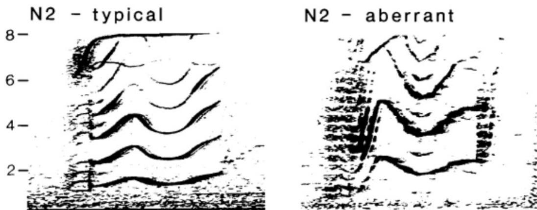
Figure 5 : Sonagramme d'un appel stéréotypé et d'une de ses formes aberrantes. Source : Ford, J., Acoustic behaviour of resident killer whales ( Orcinus orca ) off Vancouver Island, British Columbia, Canadian Journal of Zoology , janvier 1989, p. 731
