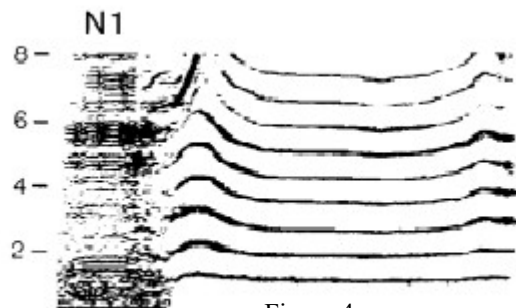
Figure 4 : sonagramme d'un appel
