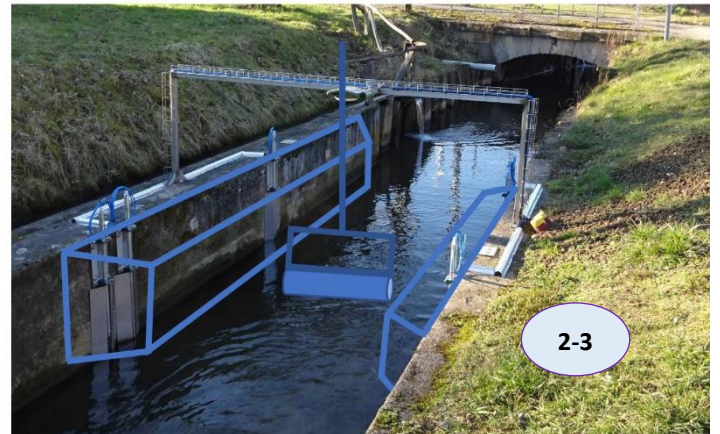
1. Vanne de la PE de la Largue (Friesen) – Etranglement et Cylindre Oscillant
