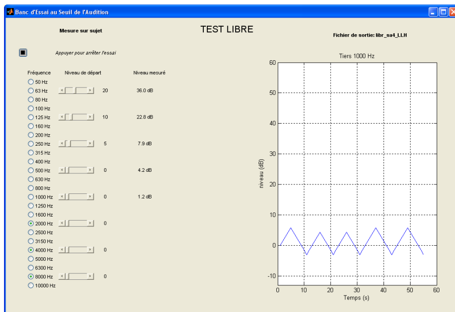
Figure 2: Exemple de résultat de détection du seuil de l'audition oreille ouverte à 1000hz
