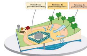
Figure 1 : Les différents PPC, ici dans le cas d'un forage (source : SE Solron)
