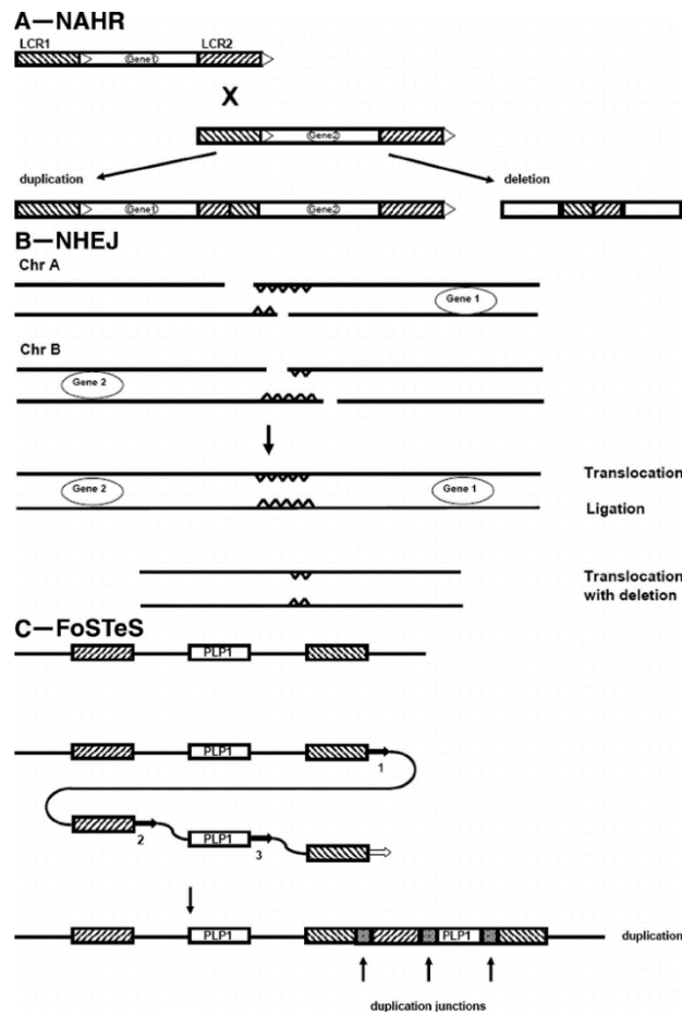
Figure 4 : Mécanismes de formation des CNV: Kalman et al. (2009) (22)
