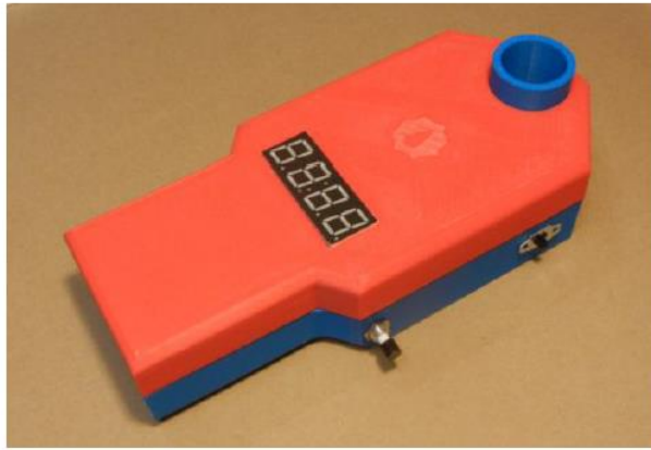
Figure 3 : Sonde de turbidité open-source proposée par Christopher D. Kelley et al., 2014
