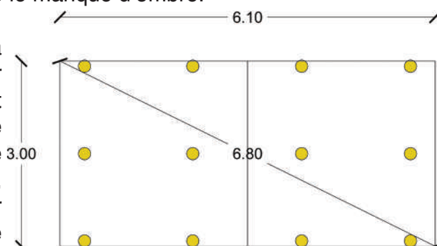
Fig 16: Schéma de tous les pilotis
