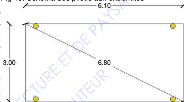
Fig 15: Schéma des pilotis aux extrémités
