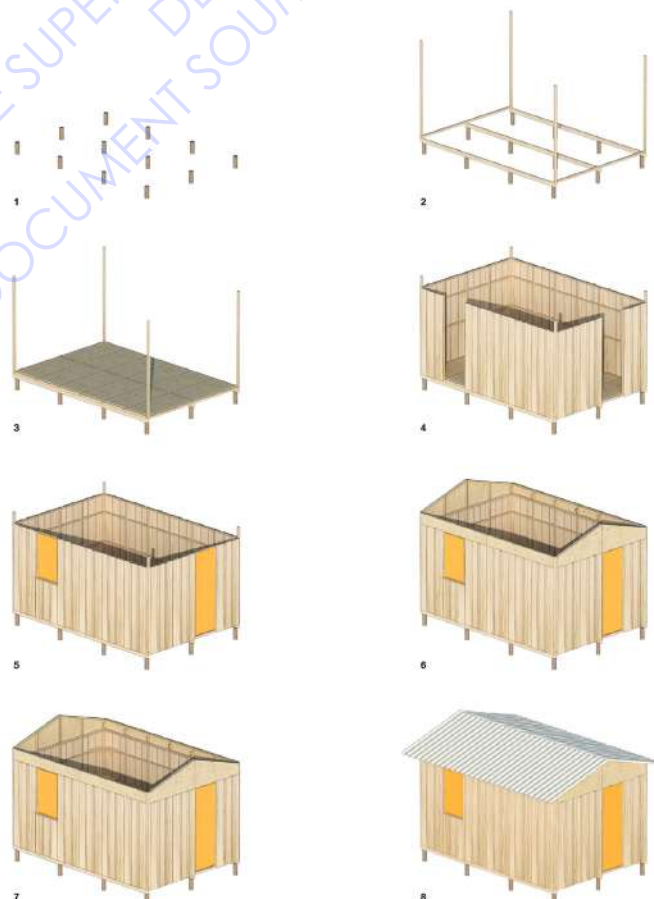
Fig 10: Manuel d'instruction du montage de l'habitat d'urgence
