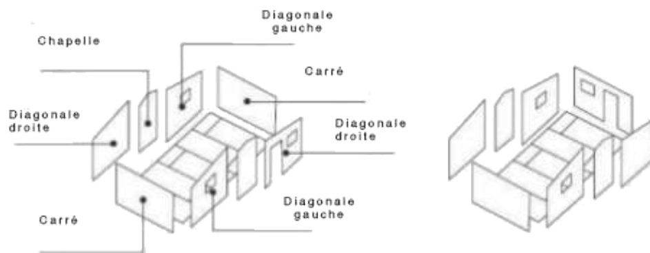
Fig 17: Schéma de construction et d'assemblage des maisons
