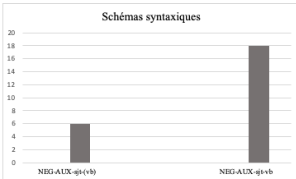
Figure 17 : Schémas syntaxiques
