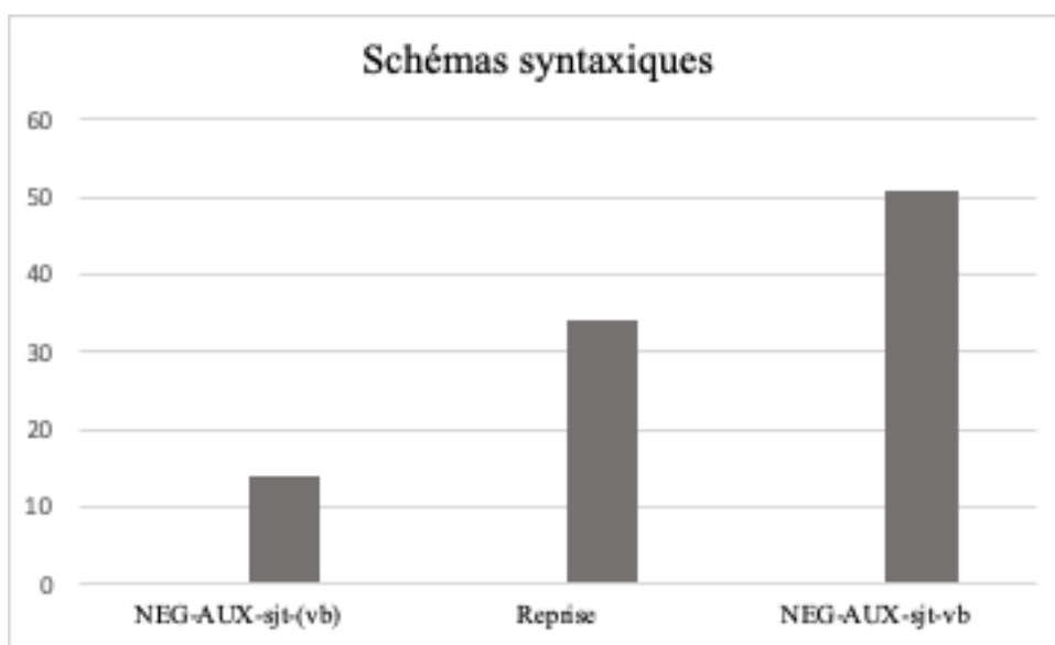
Figure 15 : Schémas syntaxiques
