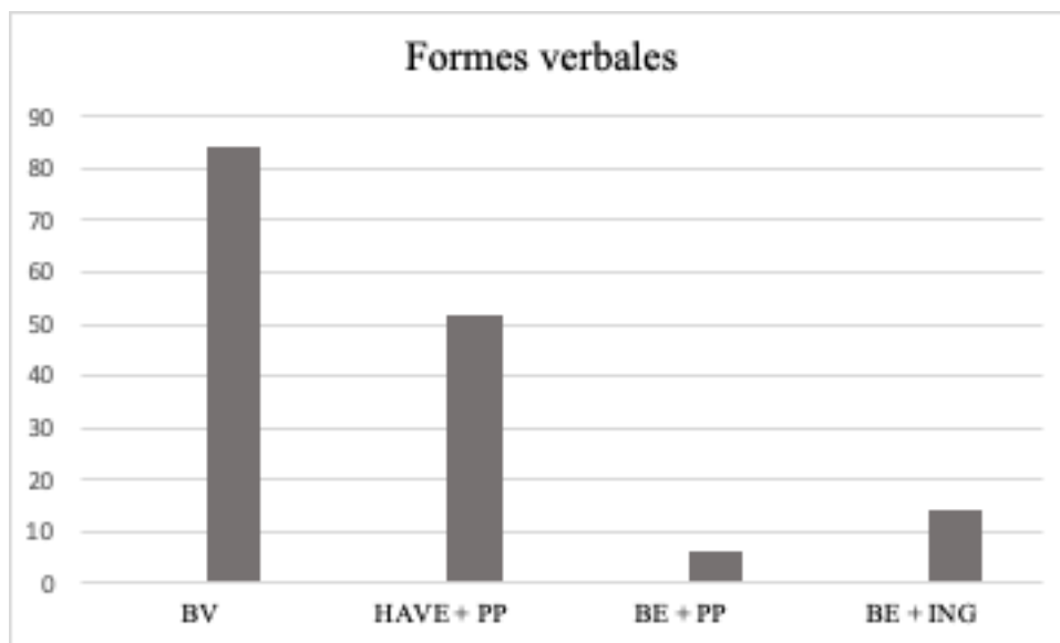
Figure 6 : Formes verbales
