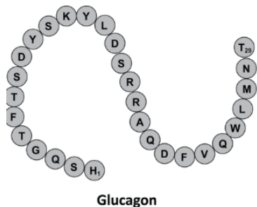
Figure 3 : Structure primaire d'une molécule de glucagon [16]
