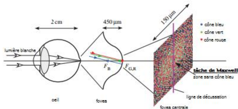
Figure 3 : Schéma de la dispersion chromatique dans la fovéa centrale.
