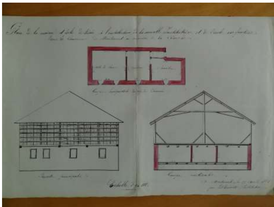
Figure 12 : Plan de l'école aux Lindarets
