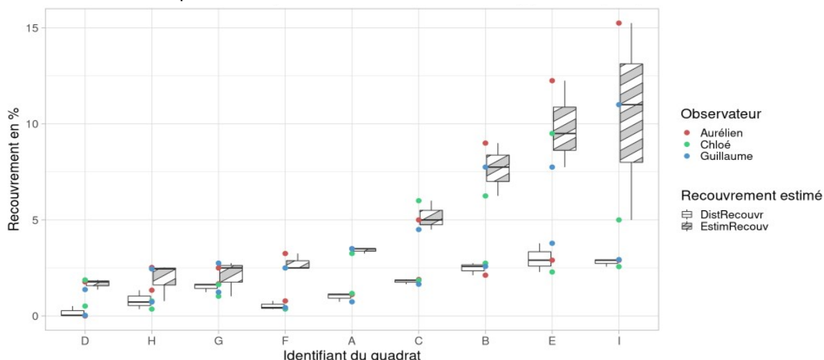
Figure 9 : Variabilité des valeurs de recouvrement obtenues par 3 observateurs sur 9 quadrats (A à I). Les valeurs de recouvrement sont obtenues grâce à deux méthodes : recouvrement estimé à partir de mesures de distances (DistRecouvr) et recouvrement estimé à vue (EstimRecouvr).
