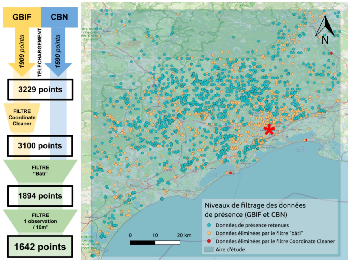
Figure 2 : Filtrage des données de présence utilisées pour les SDM à très haute résolution du thym. Montpellier est localisé par l'étoile rouge. (source personnelle)
