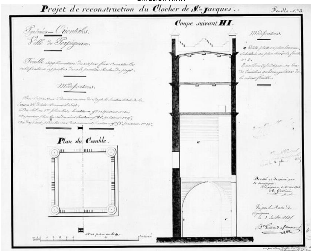
Figure 21 : Projet de reconstruction du clocher de l'église
