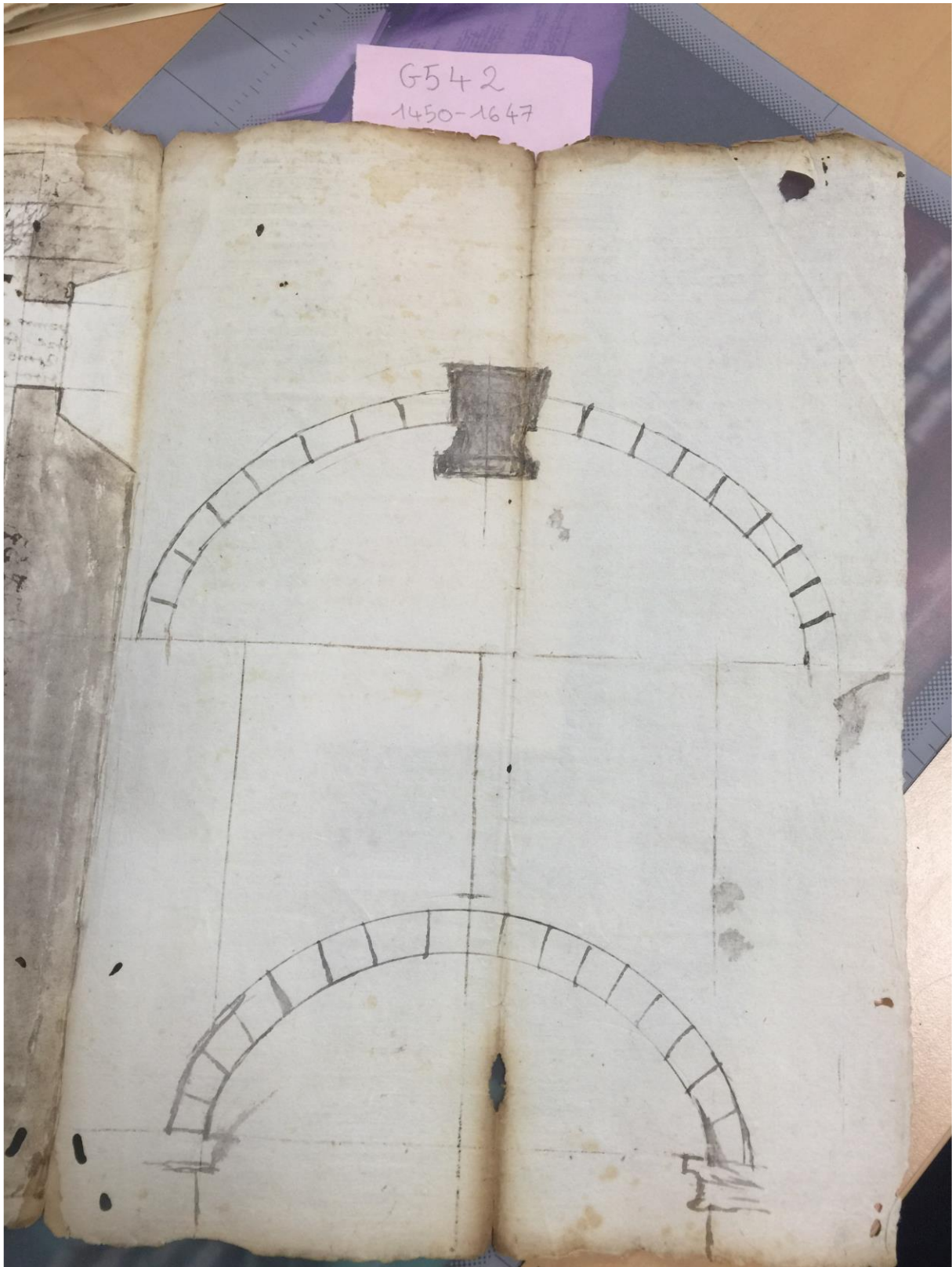
Figure 19 : Plans des voûtes de l'église Saint-Jacques
