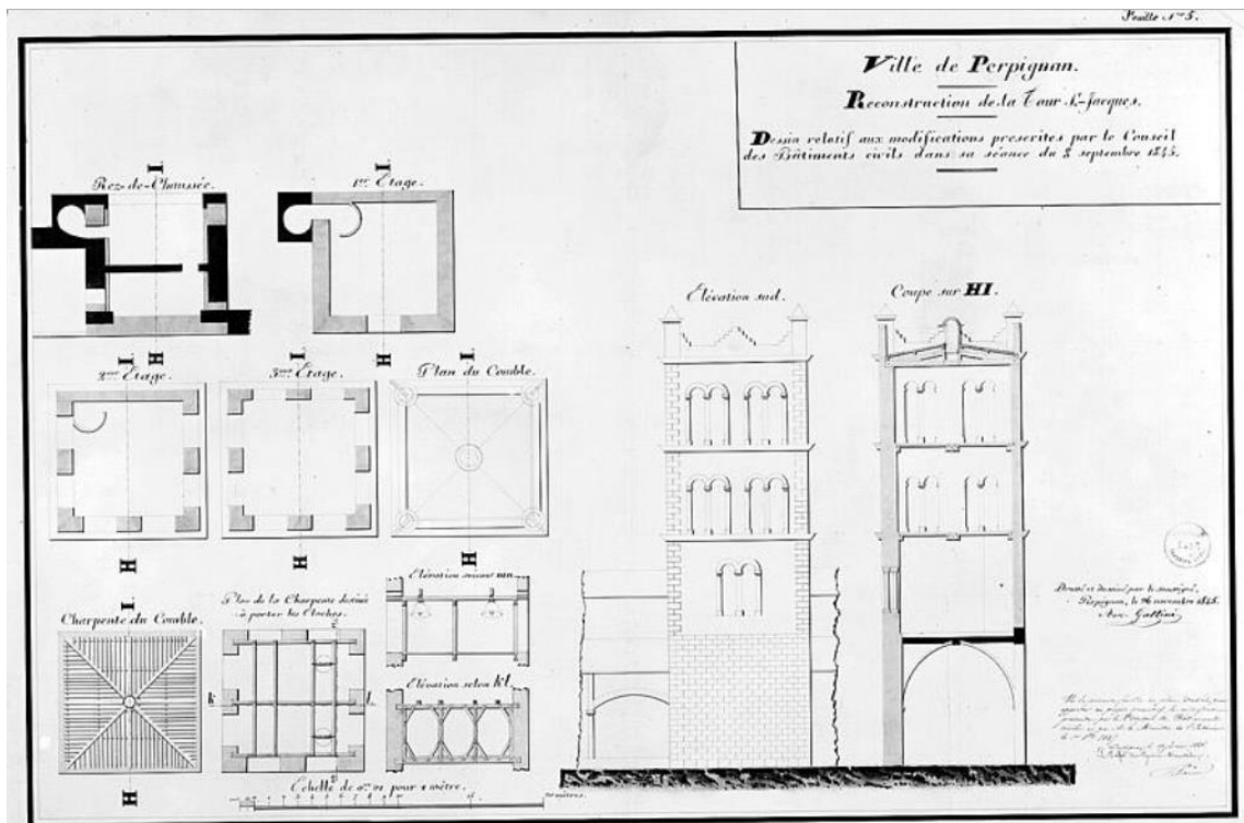
Figure 22 : Plan de reconstruction de la tour de l'édifice
