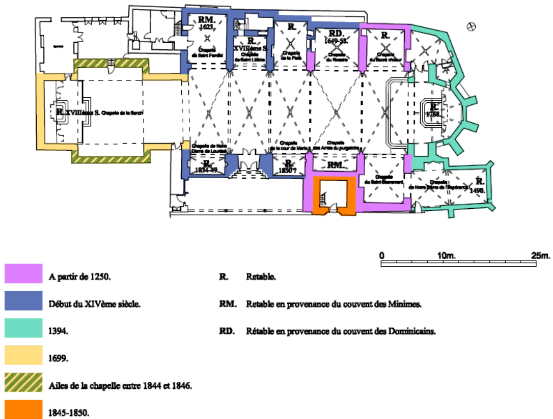
Figure 6 : Datation des différentes parties de l'église Saint-Jacques de Perpignan, plan de la DRAC de Montpellier
