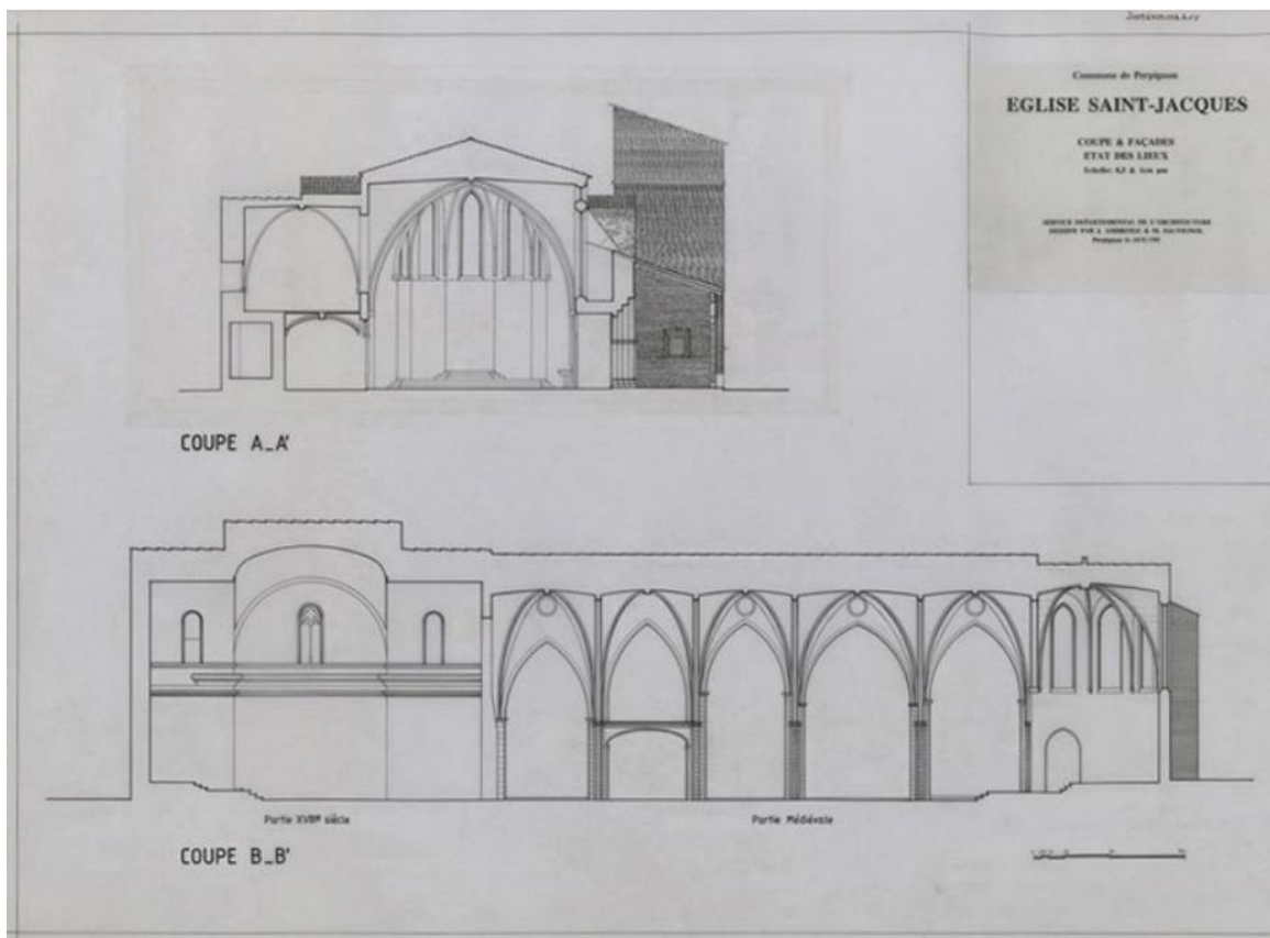
Figure 7 : Coupes transversales
