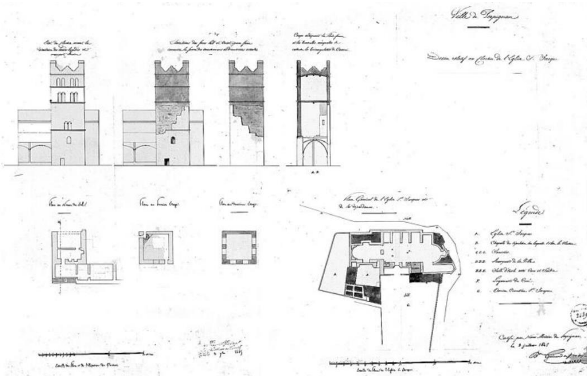
Figure 20 : Plans du clocher de l'église
