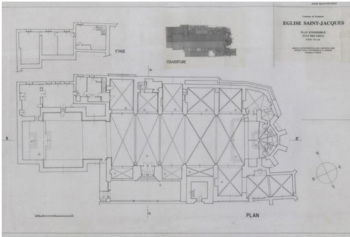
Figure 13 : Plan au sol de l'église Saint-Jacques
