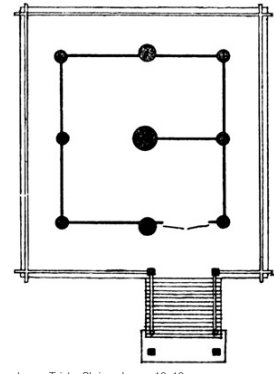
Izumo Taisha Shrine, Japan, 12x12 m.
