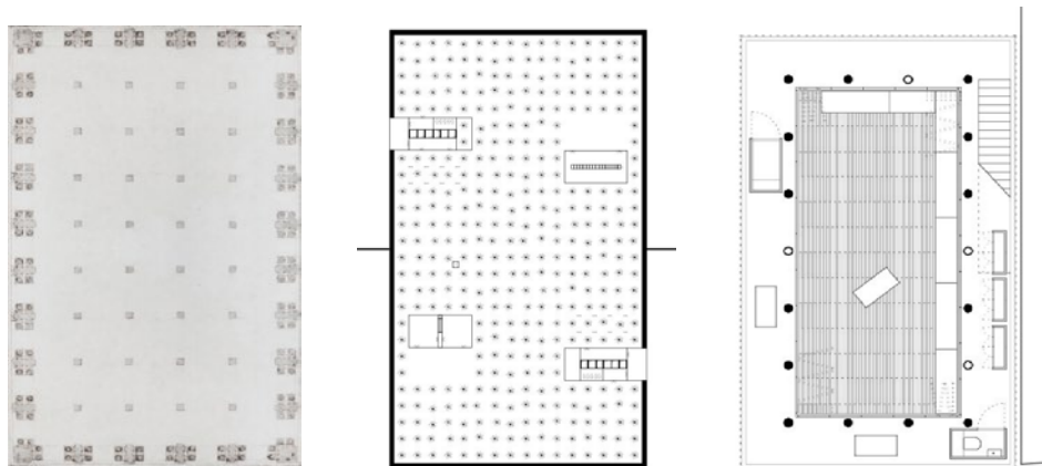
fig. 10 : Pour l'exposition Besides History, ces 3 projets ont été présentés à pied d'égalité - Palladio, Basilica, Vicenza, 1750 - Office, BORDER GARDEN, Juarez + El Paso (Mexique+USA), 2005 - MUSIC CENTER, Muharraq (Bahrain), 2016
