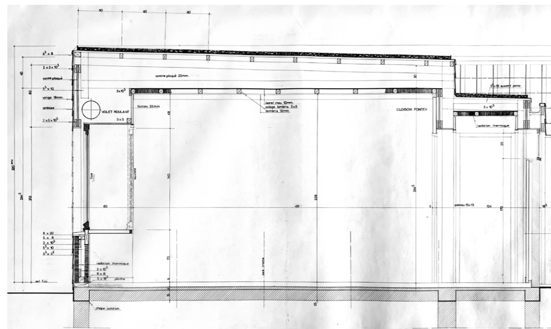
Coupe de la Maison L - Vannes
