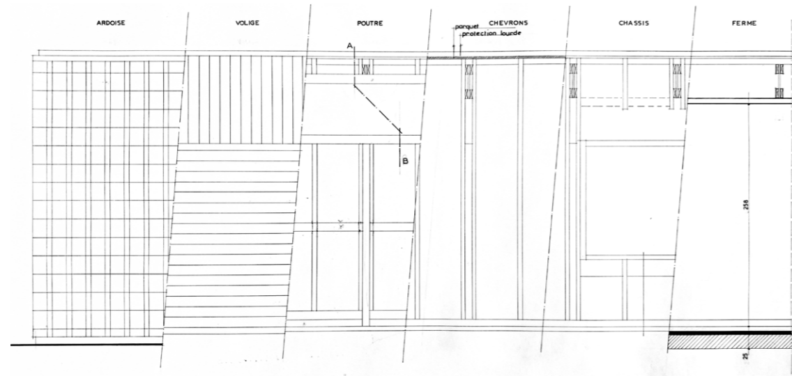
Détail de la paroi de la Maison L - Vannes
