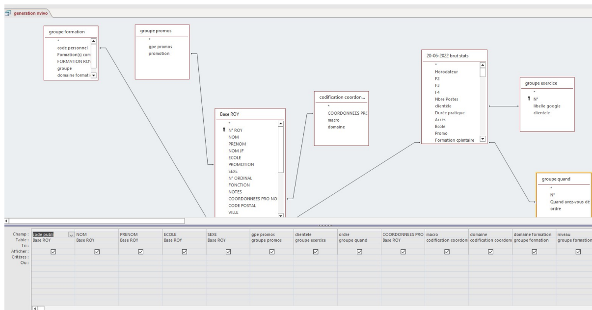
Figure 3 : Copie d'écran d'une requête Access pour générer un fichier d'attributs pour Nvivo
