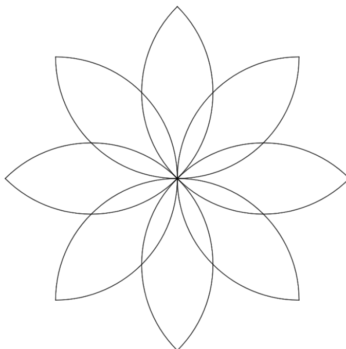
Figure 2 : Rosace à huit pétales
