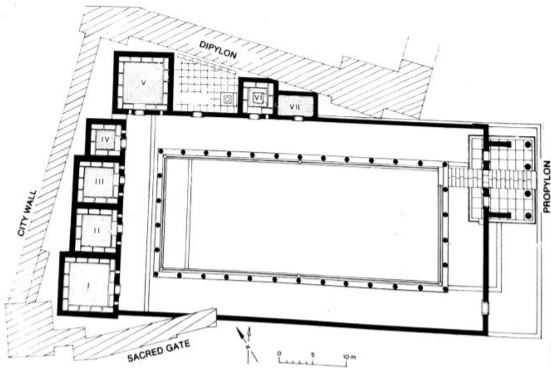
Figure 1. Plan du Pompéion d'Athènes, d'après KNIGGE 1991, p.80.
