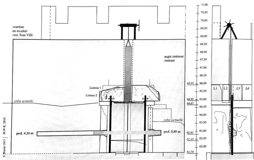
Figure 4. Restitution de la porte de Parménion, face interne et vue latérale, d'après GRANDJEAN 2011, p.530.
