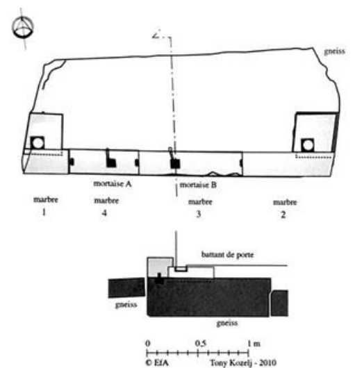
Figure 3. Restitution du seuil de la porte du Silène dans sa troisième phase (deuxième moitié du IV e siècle), d'après GRANDJEAN 2011, p.534.
