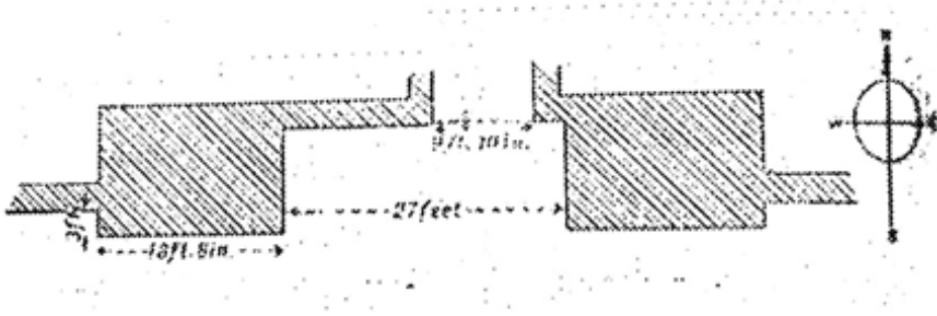
Figure 1. Plan de la porte A d'Abai (v e siècle), d'après TYPALDOU-FAKIRIS 2004, p.133.
