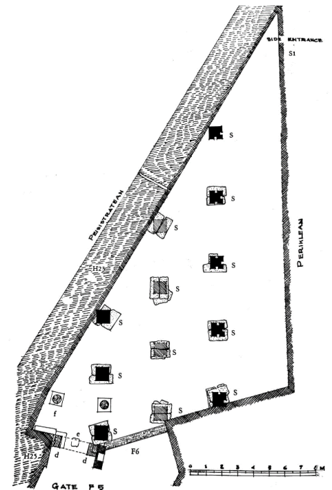
Figure 3. Plan du secteur de la porte F5 d'Éleusis, d'après MYLONAS 1969, fig.36.
