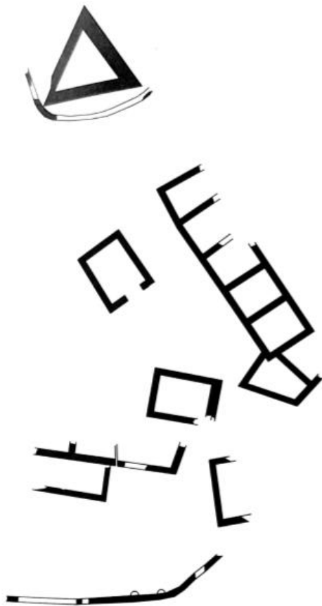
Figure 1. Plan du secteur de l'Hérôon au sud de la Porte Ouest d'Érétrie vers le milieu du VIe siècle, d'après BERARD 1970, p.175.
