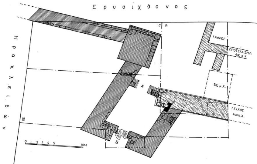
Figure 1. Dessin des restes de la porte du Pirée, d'après TRAVLOS 1988.
