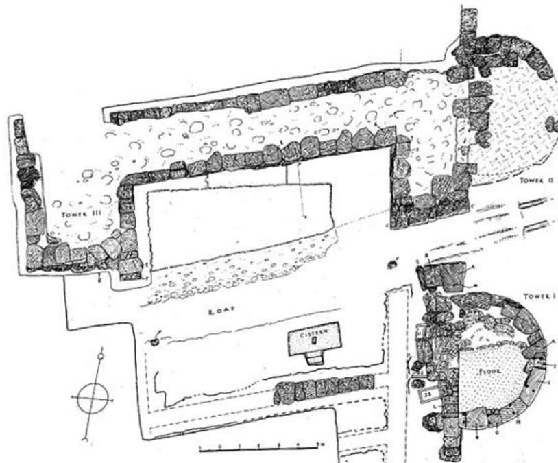
Figure 2. Plan de la porte isthmienne de Corinthe, d'après WINTER 1974, p.224.
