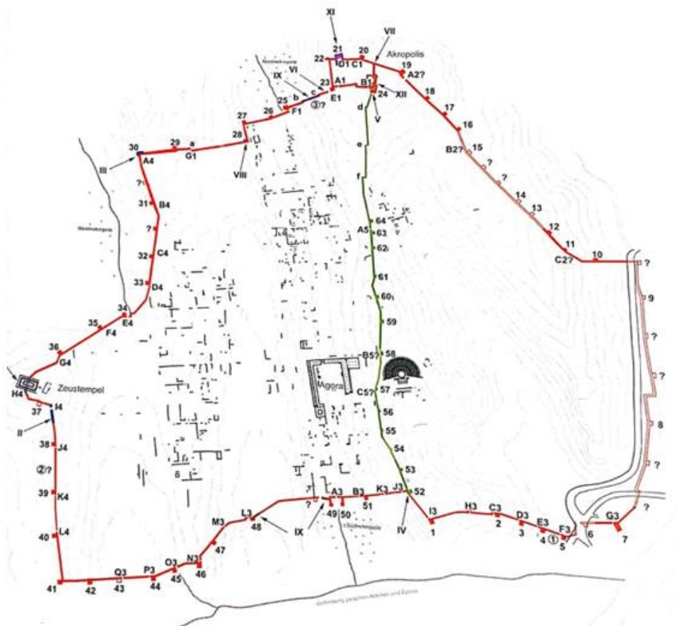
Figure 1. Plan de la fortification de Stratos (entre le Ve et le IVe siècle), d'après MÜTH 2016, p.342.
