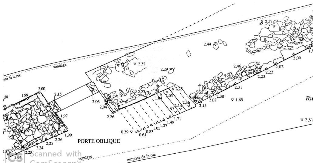
Figure 3. Plan de la porte oblique et de son escalier, d'après GRANDJEAN 2011, p.285.
