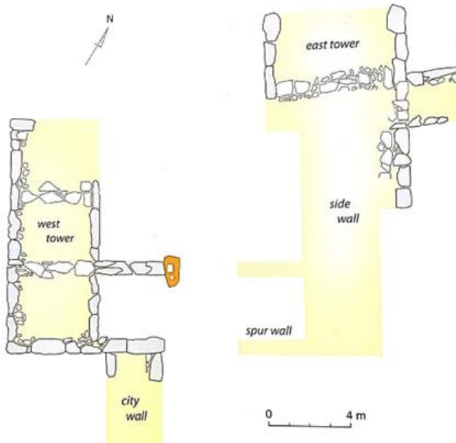
Figure 1. Plan de la porte Nord-Ouest de Néa Halos, d'après REINDERS 2014, p.49.
