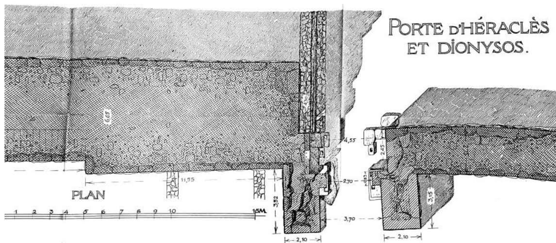
Figure 3. Plan d'ensemble et élévation de la porte d'Héraclès, d'après PICARD 1962, p.
