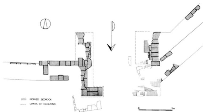
Figure 2. Plan de la porte nord de Goritsa, d'après BAKHUIZEN 1992, p.114.
