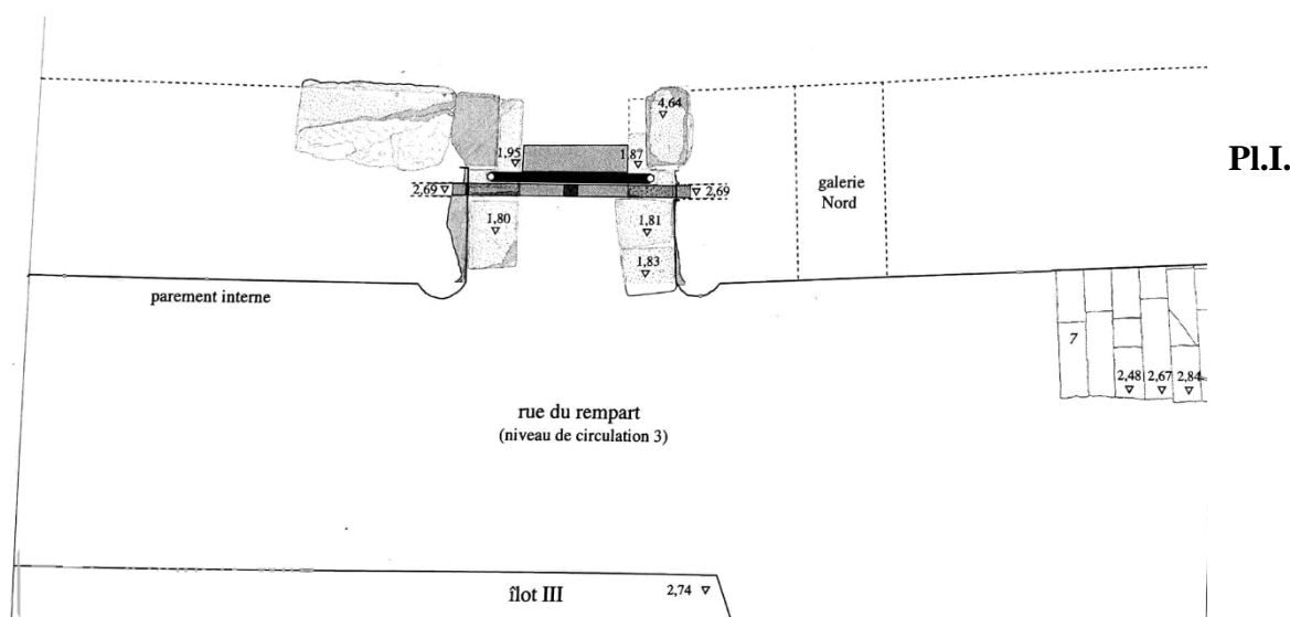
Figure 7. Restitution de la porte d'Hermès vue du dessus, d'après GRANDJEAN 2011, p.526.
