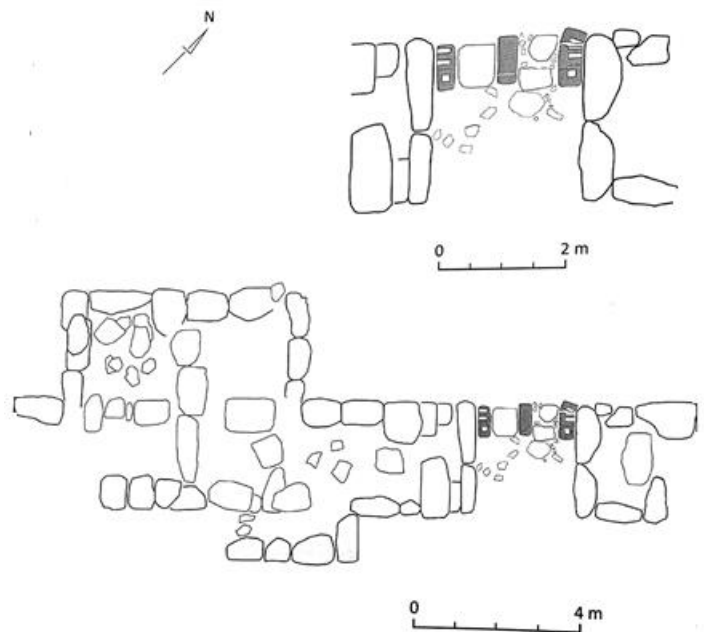
Figure 2. Plan du seuil de la porte de l'acropole de Néa Halos, d'après REINDERS 2014, p.54..
