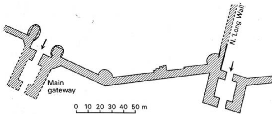
Figure 2. Plan des portes nord de l'enceinte du Pirée, d'après LAWRENCE 1979, p.307.
