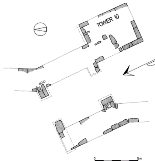
Figure 3. Plan de la porte est de Gortisa, d'après BAKHUIZEN 1992, p.103.
