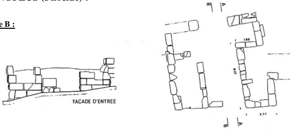
Figure 1. Porte B de Panopeus en Phocide, à gauche l'élevation depuis l'extérieur, à droite le plan du passage au sol, d'après TYPALDOU-FAKIRIS 2004, p.179.
