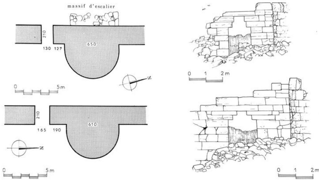
Figure 1. Poternes à l'est de l'enceinte de Phigalie, plan et restitution de l'élévation, d'après ADAM 1982, p.93.
