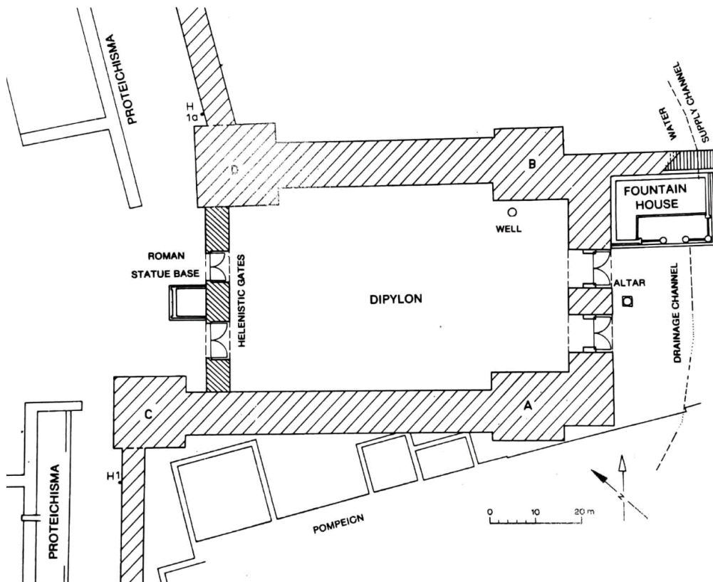
Figure 2. Plan du Dipylon d'Athènes à l'époque hellénistique/romaine, d'après KNIGGE 1991, p.71.
