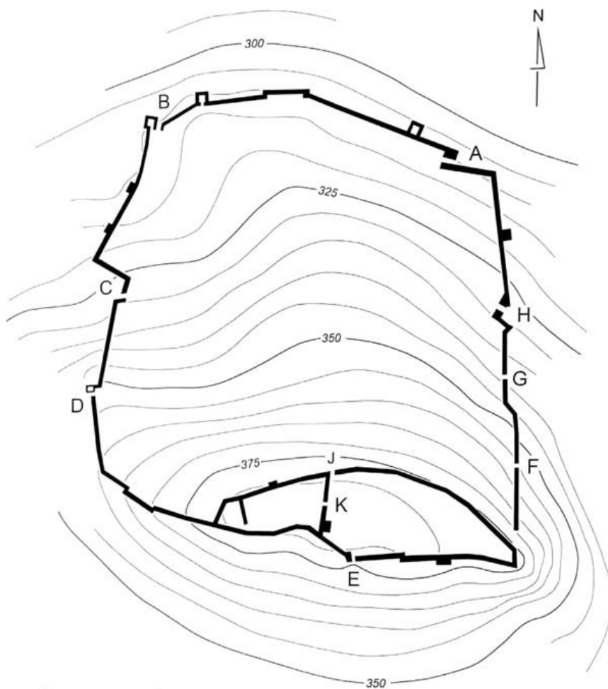
Figure 1. Plan de l'enceinte d'Érétrie de Thessalie, fortifications probablement édifiées à la fin du IV e siècle, d'après REINDERS 2014, p.124.
