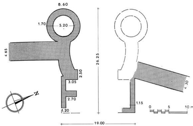
Figure 3. Plan de la porte A de Mantinée, d'après ADAM 1981, p.89.
