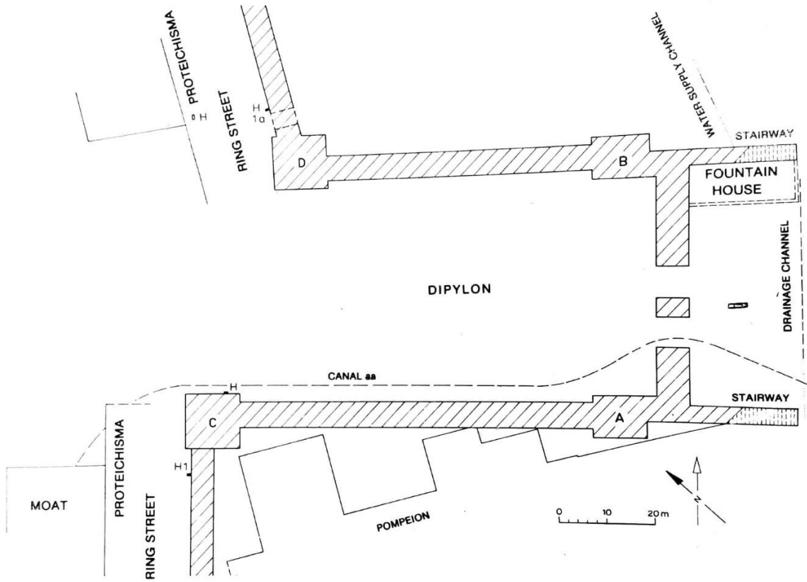
Figure 1. Plan de du Dipylon d'Athènes entre 479 et 307, d'après KNIGGE 1991, p.72.
