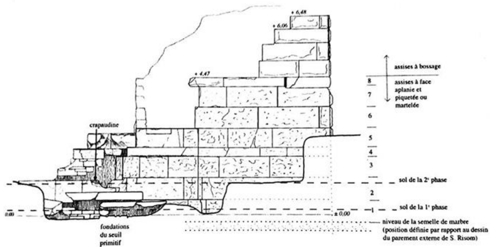
Figure 2. Coupe de l'élévation latérale de la porte et des niveaux de sol, d'après GRANDJEAN 2011, p.225
