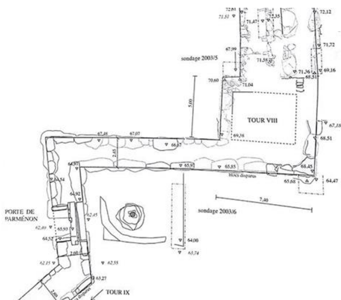
Figure 8. Plan de la fortification de Thasos au niveau de la porte de Parménion et de la tour de protection, d'après GRANDJEAN 2011, p.134.
