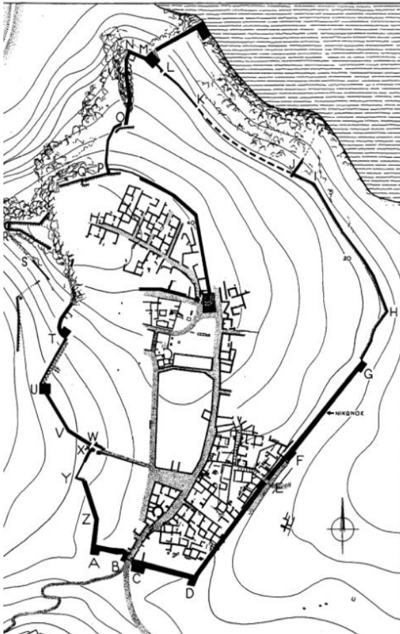
Figure 1. Plan des fortifications de Rhamnonte, d'après PETRAKOS 1997, fig.2.
