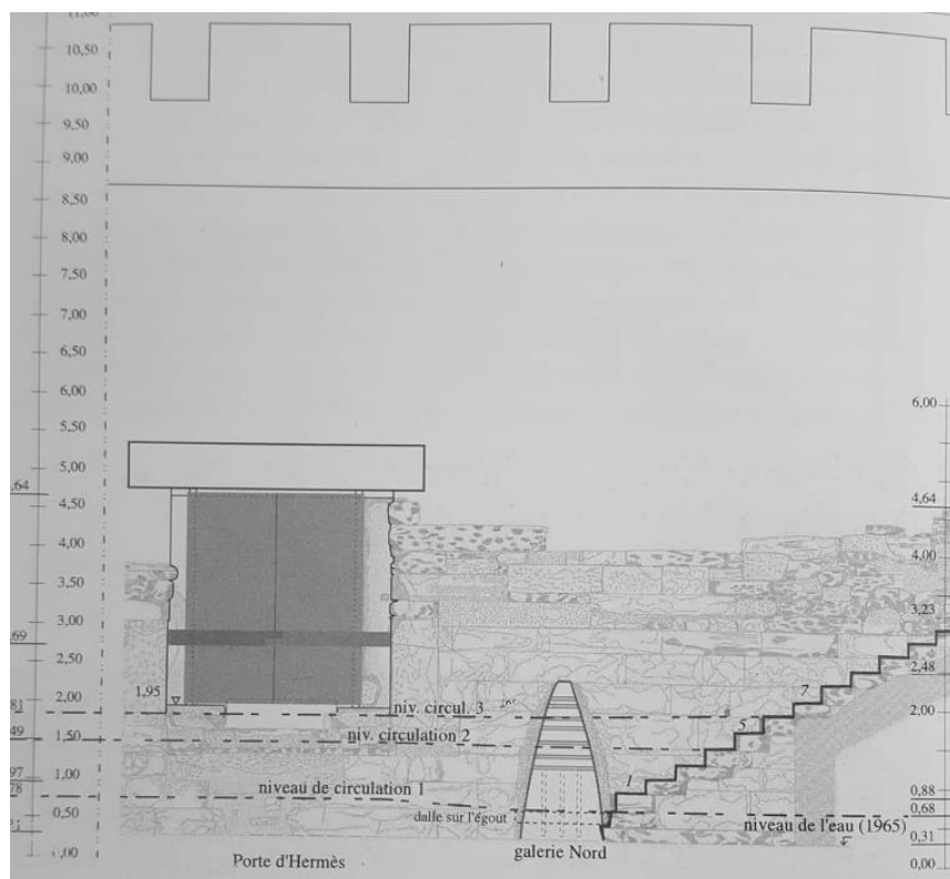
Figure 3. Restitution de la porte d'Hermès dans ses trois premières phases, d'après GRANDJEAN 2011, p.526.
