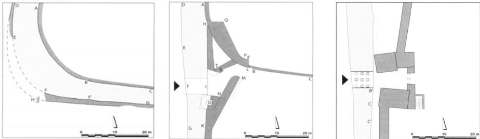
Figure 1. (Au-dessus) Plans de la porte ouest et de son secteur, à l'époque géométrique (gauche), l'époque archaïque (centre) et classique (droite), FACHARD 2004, p.94, 95 et 99.
