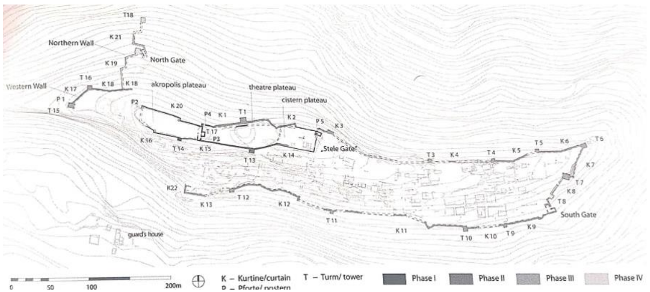
Figure 2. Plan des fortifications de Platiana (fin du IVe siècle – début IIIe), d'après MÜTH 2016, p.313.
