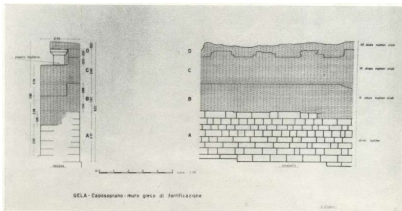
Figure 2. Restitution de l'élévation du mur de Timoléon à Géla, on y voit le socle (A) et les couches successives de briques (B = couche originelle), d'après ADAMESTEANU 1957, p.38.
