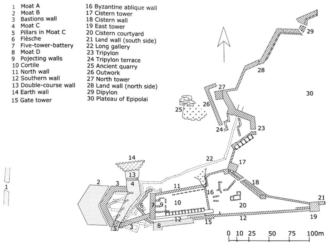
Figure 2. Plan du secteur du château de l'Euryale et détail des structures.
