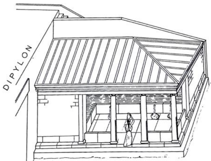
Figure 3. Restitution de l'élévation de la fontaine du Dipylon, d'après KNIGGE 1991, p.75.
