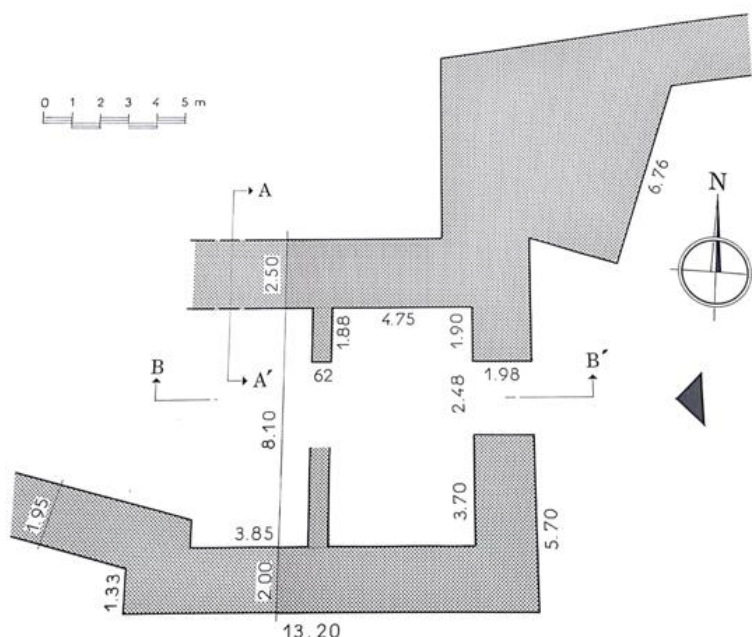
Figure 1. Plan de la forteresse d'Eleuthères (Ve ou IVe siècle), d'après ADAM 1982, p.216.
