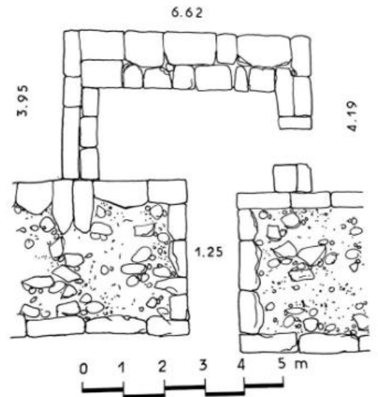
Figure 4. Tour de l'enceinte de Mantinée avec sa poterne creusée dans le flanc, d'après FOUGERES 1989, p.159.
