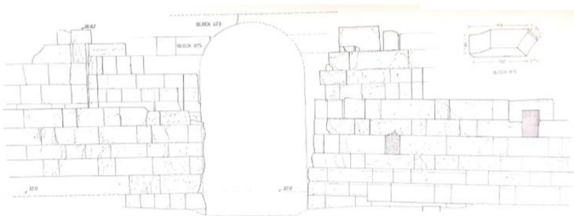
Figure 3. Proposition de restitution de l'élévation de la porte Nord de Sélinonte, d'après MERTENS 2003, p.103.
