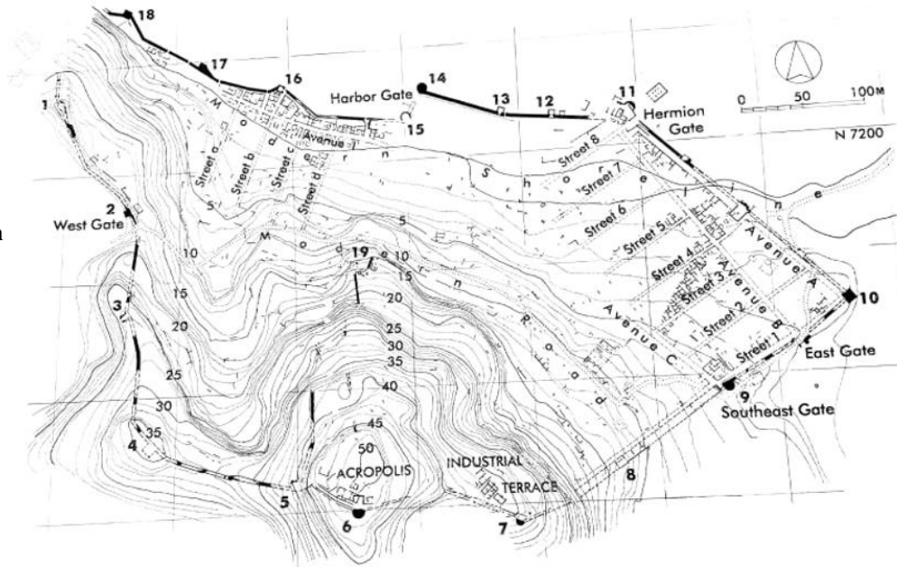
Figure 1. Plan de la ville et la fortification d'Halieis (époque classique), d'après MCALLISTER 2005, fig.18.
