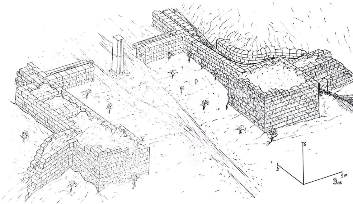
Figure 1. Restitution de la porte sud de Messène, d'après MÜTH 2010, p.120.
