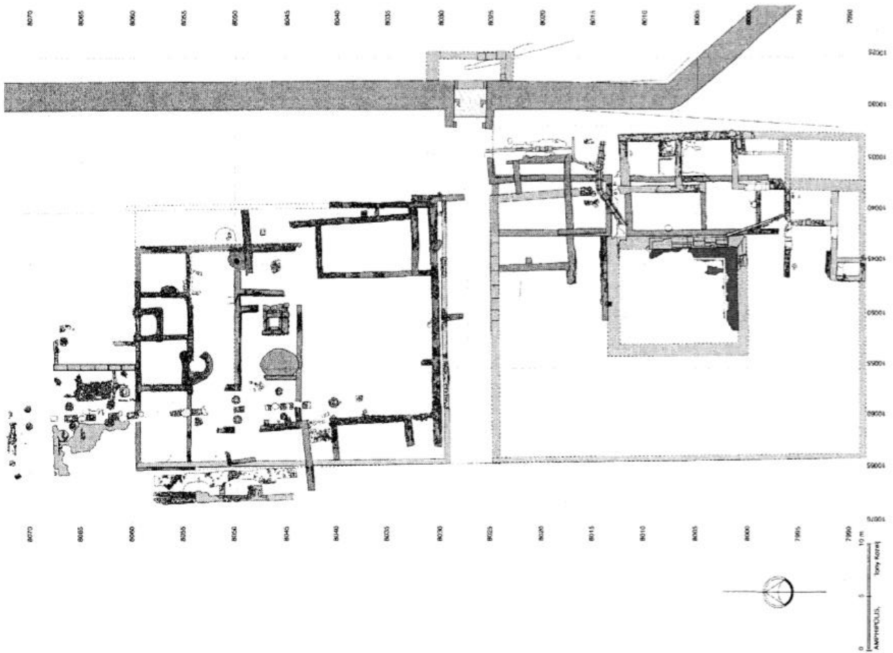
Figure 1. Plan du secteur de la porte Est et de sa tombe, d'après KOUKOULI-CHRYSANTHAKI 2002, p.61.
