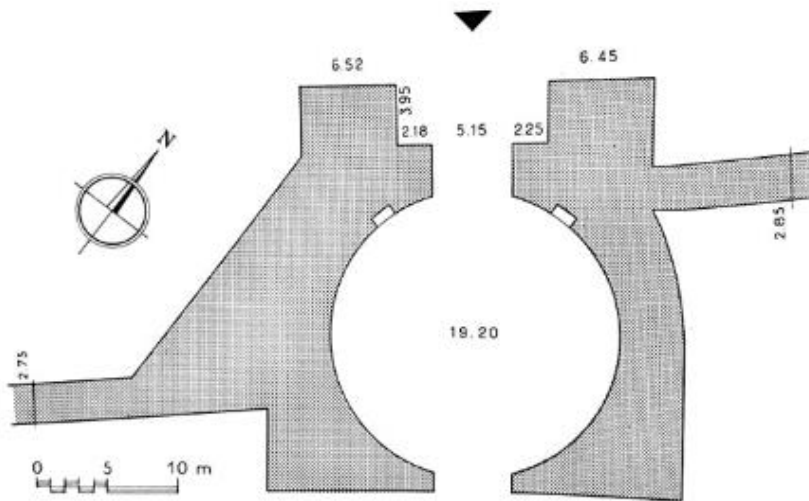
Figure 1. Plan de la porte à cour dite d'Arcadie (IVe siècle ou début IIIe), d'après ADAM 1982, p.90.
