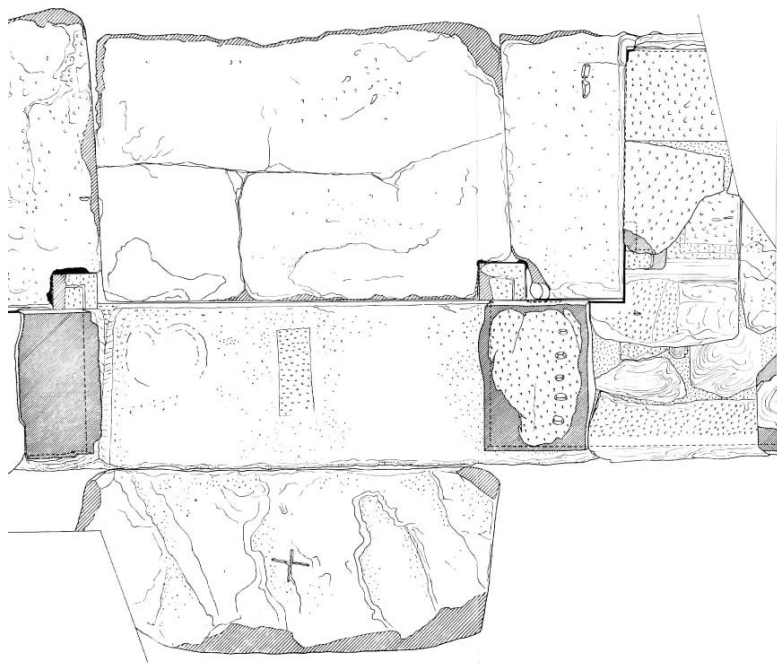
Figure 3. Dessin du seuil de la porte au char, d'après PICARD 1962, p.114-115 (fig.48).
