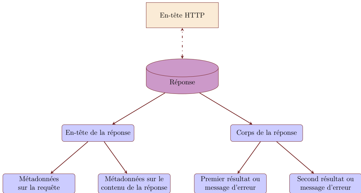
FIGURE 9.1 – Modèle de réponse renvoyé par KatAPI
