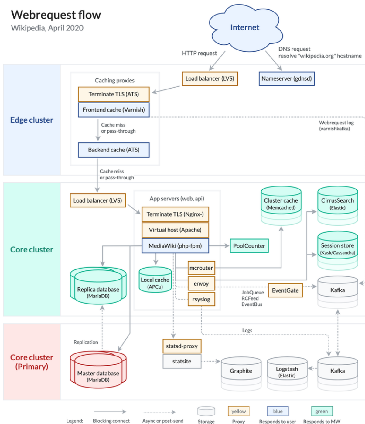
FIGURE F.1 – L'architecture des bases de données de la Wikimedia Foundation (schéma réalisé par Timo Tjihof en 2020, disponible dans le domaine public avec la licence Creative Commons CC0.1.0 Universal Public Domain License)
