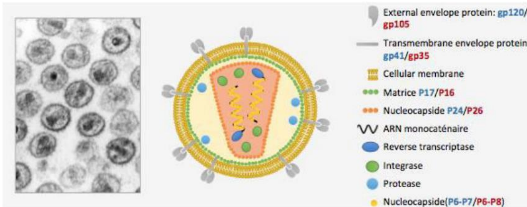
Figure 2. Structure de la particule virale VIH. Le nom des protéines virales de structure et d'enveloppe (donné en fonction du poids moléculaire de la protéine) est indiqué en bleu pour le VIH-1 et en rouge pour le VIH-2.
