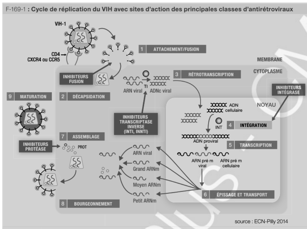
Figure 2 : Représentation schématique du cycle de réplication du VIH
