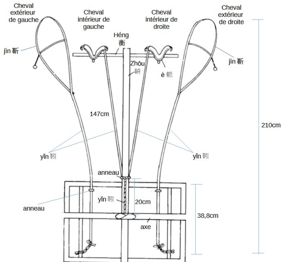
Figure 56: Disposition des yǐn des quatre chevaux attachés à la plateforme du char no. 1 du Mausolée du Premier Empereur de Qín
