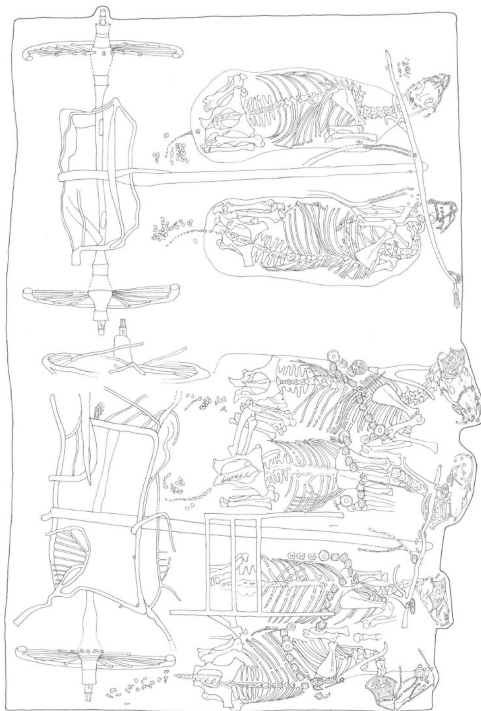
Figure 106: Fosse de char avec leurs chevaux découverte à Zhāngjiāpō de Cháng'ān xiàn dans le Shǎnxī (no. 168)
