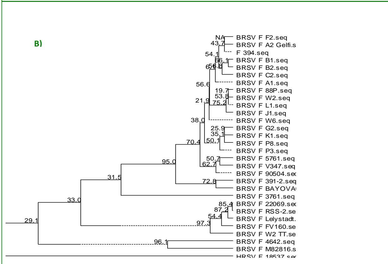
Figure 16 : Arbres phylogénétiques sur la séquence nucléotidique de F (position nucléotidique 512-1254 ) entre les souches 3761, A2-Gelfi et W2 en comparaison avec les séquences d'isolats de VRSB obtenus à partir des banques de données. (Programme MegAlin, DNASTar Lasergen, alignement multiple par le programme CLUSTAL W). A) arbre phylogénétique global, B) grossissement sur les séquences VRSB
