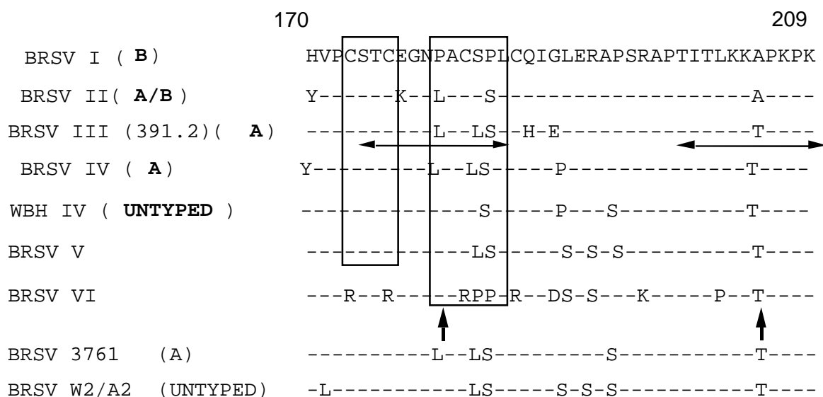
Figure 22 : Séquence consensus pour chaque sous-groupe de VRSB entre les résidus aminoacides 170 et 209 de la protéine G. Les flèches horizontales représentent les épitopes linéarisés étudiés par Langedijk et al. (1997), les flèches verticales montrent les mutations qui ont déterminé les sous-groupes d'antigènes et les rectangles indiquent la localisation des hélices \alpha . Les séquences des souches 3761 et W2 ont été ajoutées.
