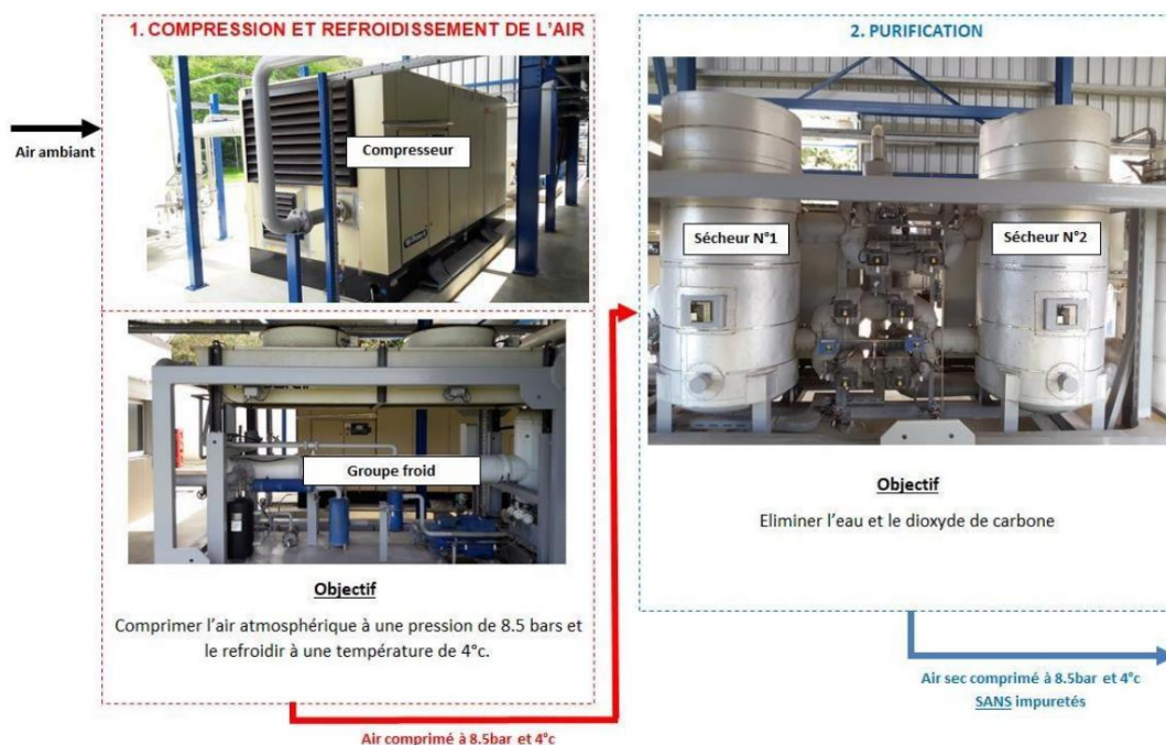
Figure 6: Etapes de compression, refroidissement, et purification de l'air dans le processus de cryodistillation.
