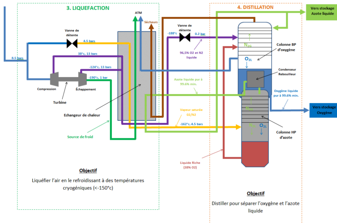
Figure 7: Etapes de liquéfaction, distillation dans le processus de cryodistillation.
