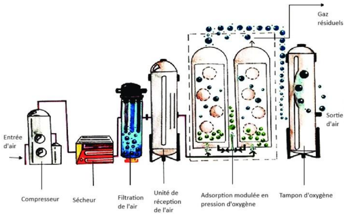
Figure 9 : Schéma d'un système PSA (type production industrielle).
