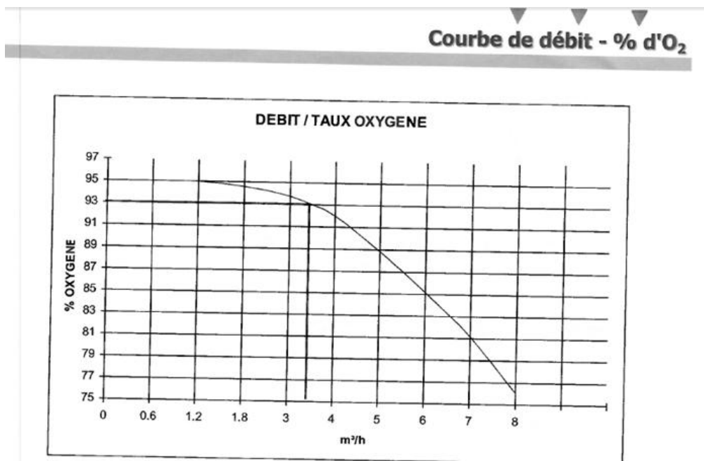
Figure 16: Débit d'oxygène en fonction de la pureté en oxygène produit les concentrateurs d'oxygène
