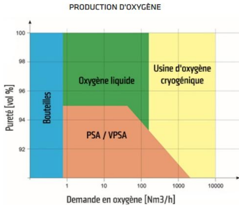
Figure 12: Pureté et demande en oxygène atteignable en fonction du concept de production
