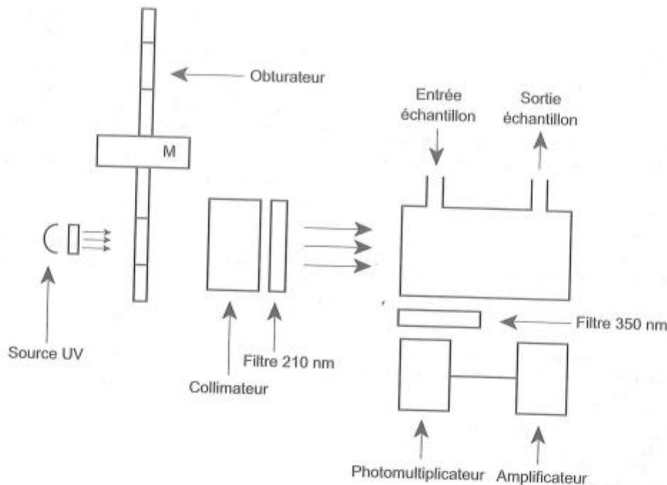
Figure 2455.-1. – Analyseur à fluorescence UV
