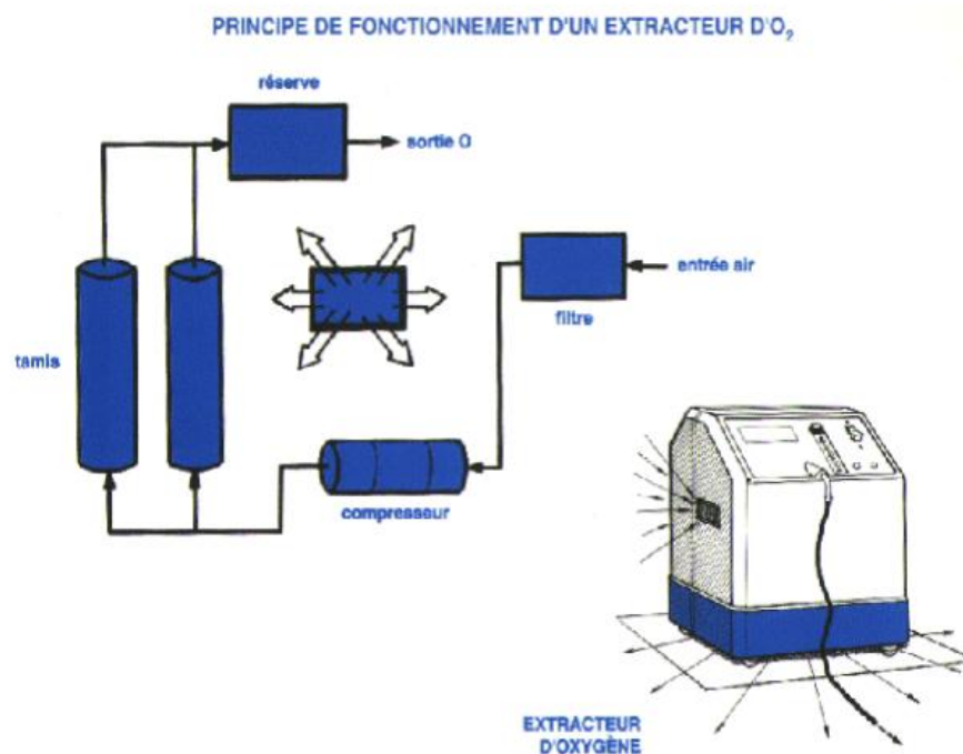
Figure 8 : Principe de fonctionnement d'un extracteur d'oxygène
