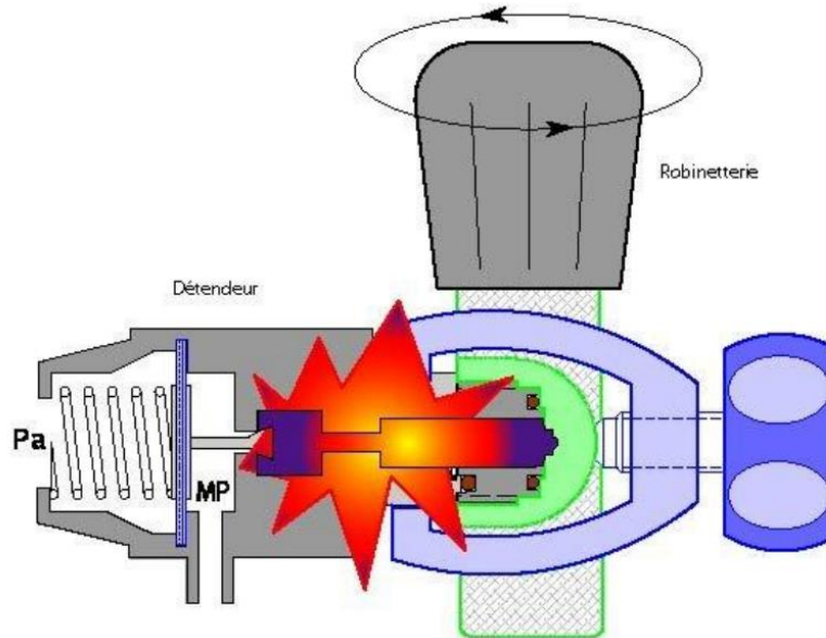
Figure 15: Déclenchement d'un coup de feu au sein du manodétendeur.
