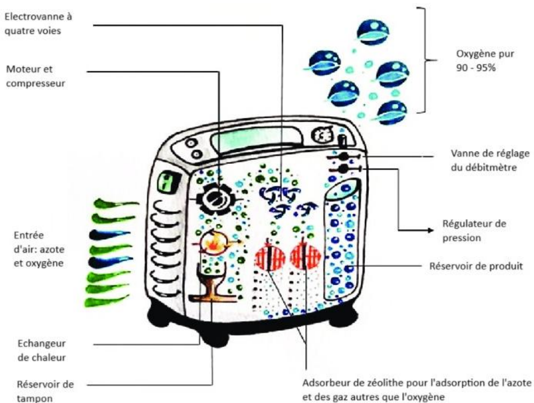
Figure 10: Schéma des différentes parties d'un concentrateur à oxygène.
