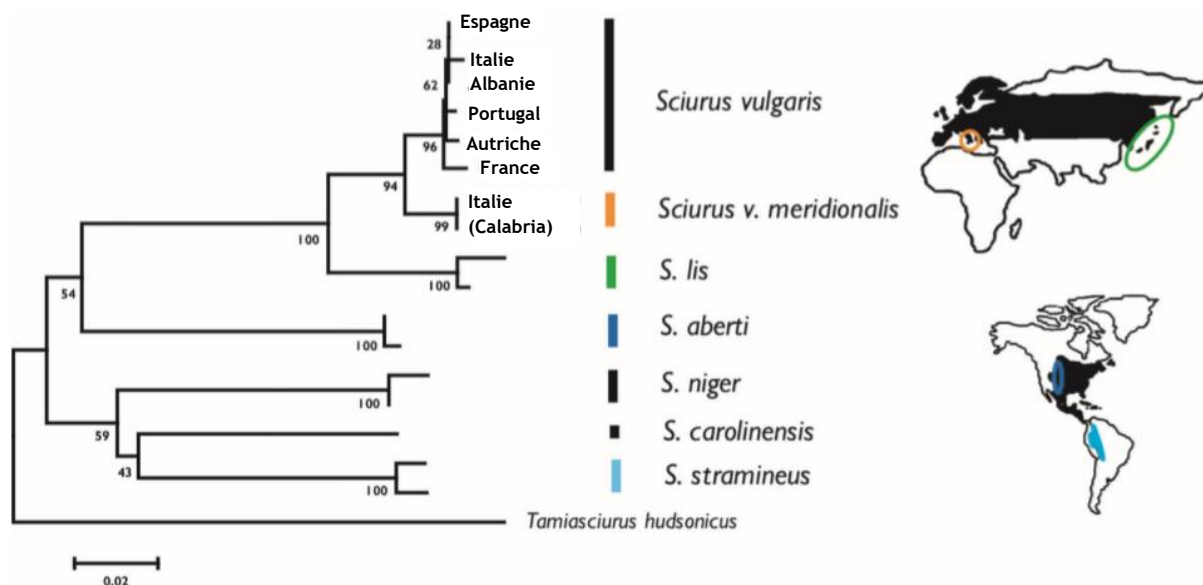
Figure 1 : Arbre phylogénétique du genre Sciurus (Grill et al. , 2009)
