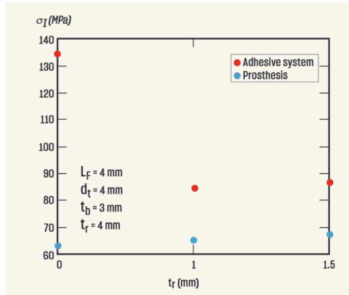
Figure 18 : contraintes emmagasinées par la prothèse (bleu) et par le système adhésif (rouge) en fonction de l'épaisseur de l'ailette (Attal et al. 2022).
