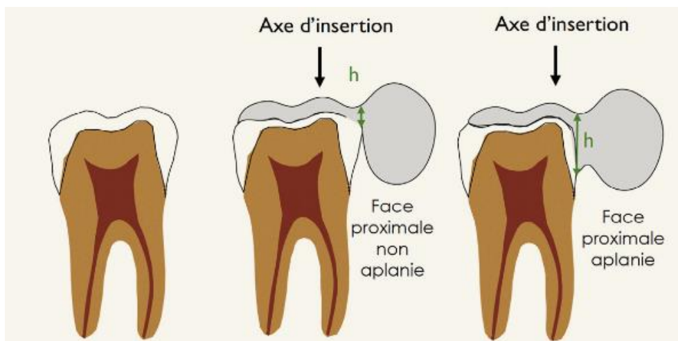
Figure 17 : schéma montrant l'aplatissement de la face proximale et son impact sur la valeur h . Ici, la préparation de droite présentera une bien meilleure résistance mécanique (Attal et al., 2022).
