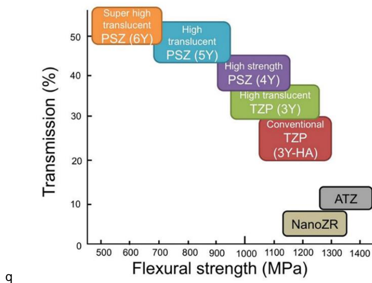
Figure 21 : graphique représentant la translucidité (ordonnée) par rapport à la résistance à la flexion des différentes zircones (abscisses) (Kongkiatkamon et al., 2023).
