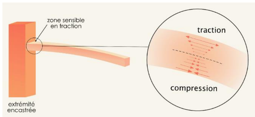
Figure 7 : illustration des forces de traction et compression appliquées sur une architecture cantilever (Attal et al., 2022).
