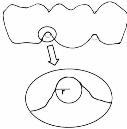
Figure 6 : représentation du rayon de courbure des connectives de bridges (Oh et Anusavice 2002)
