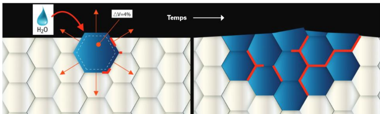
Figure 19 : illustration de la fatigue hydrique à basse température. L'eau pénètre dans la structure cristalline entraînant la formation de grains qui augmentent de volume et diminuent les propriétés mécaniques de la céramique (Mainjot, 2019)
