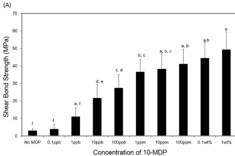
Figure 26 : lien entre la concentration de 10-MDP appliquée à la zircone et la résistance aux forces de cisaillement observées. (Nagaoka et al. 2017)
