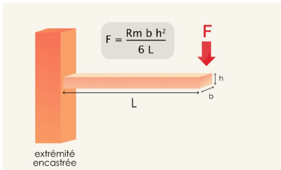
Figure 9 : schéma représentant la force que peut supporter une structure en cantilever (Attal et al. 2022)
