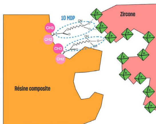
Figure 25 : schéma représentant le lien chimique permis par les molécules de 10-MDP entre la zircon et le composite de collage (Boitelle, Attal, et François 2023)
