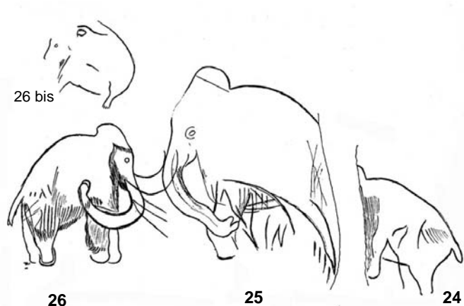
Fig. 95 – Groupe des trois mammoths n° 24, 25, 26 et du mammoth naturel 26 bis. Les n° 24 et 25 font face au n° 26. Relevé d'après H. Breuil, 1924.
