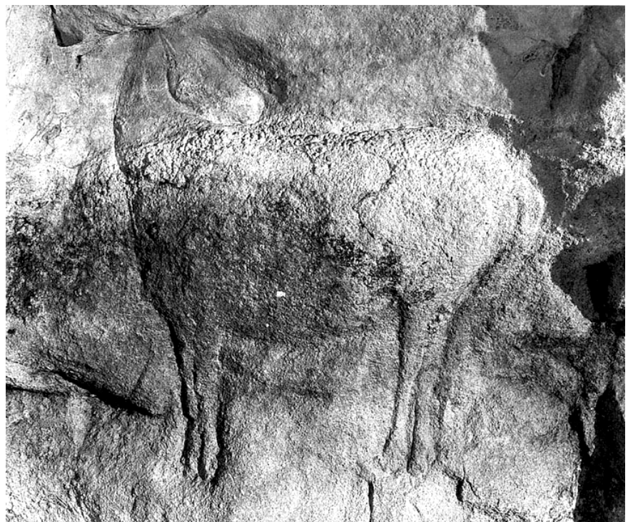
Fig. 38 – Le Roc-aux-Sorciers. Cheval tournant la tête. Photos G. Pinçon.
