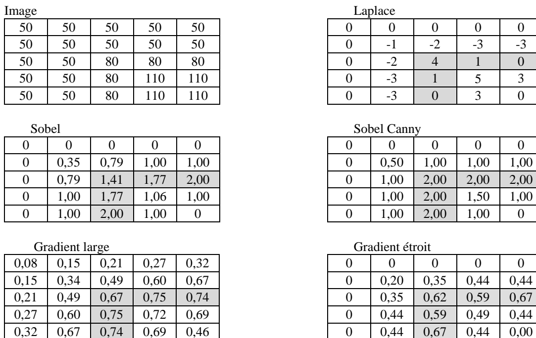
Figure 3.7 : Détection des contours en coin
