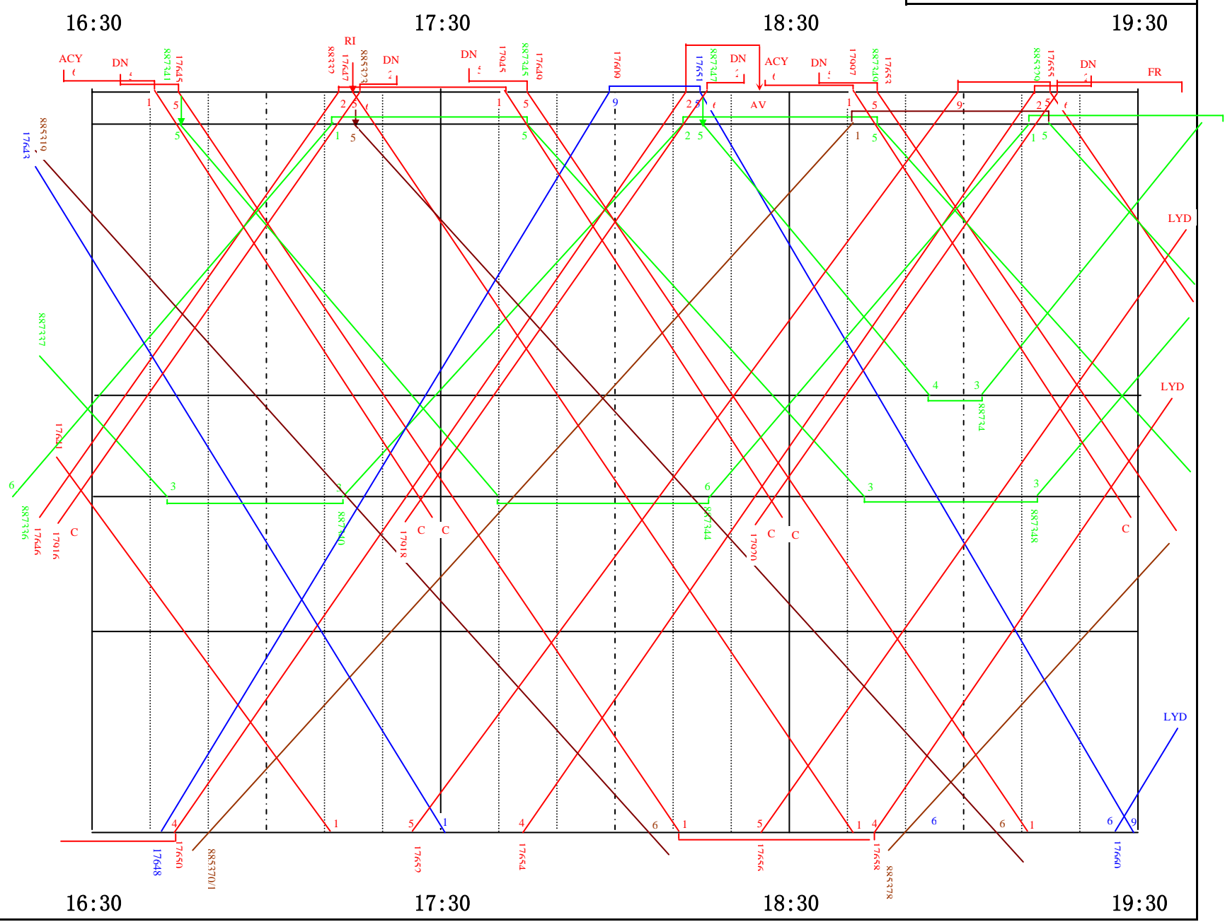
Annexe 6 - Graphique de circulation (heures de pointe)
