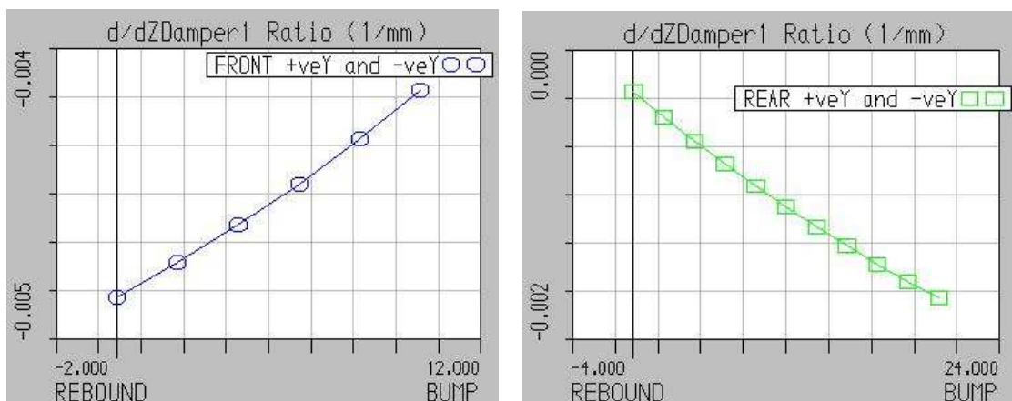
Graphique 2 : Lambda'
