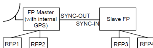
Figure 107 : Synchronisation câblée et avec GPS [dect2]
