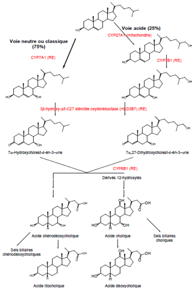
Figure 3 : Synthèse des acides biliaires, selon Lefebvre, 2009. Les acides biliaires sont formés par deux voies principales, dites classique et acide. Il existe deux voies minoritaires ayant pour substrat initial le 24-hydroxycholestérol ou le 25-hydroxycholestérol. Les acides lithocholique et déoxycholique sont dits acides biliaires secondaires. RE : réticulum endoplasmique.
