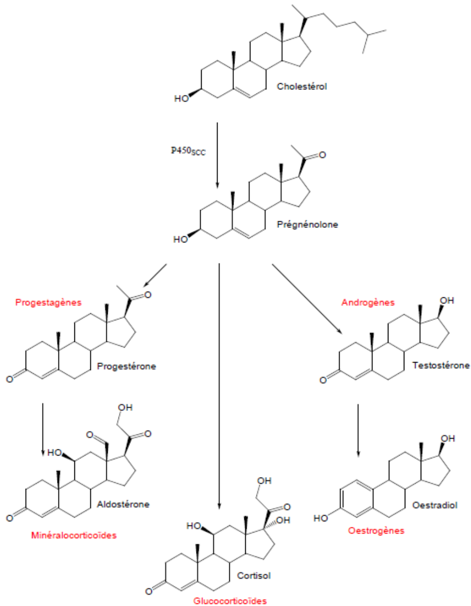
Figure 4 : Filiation et structure des hormones stéroïdiennes [3].
