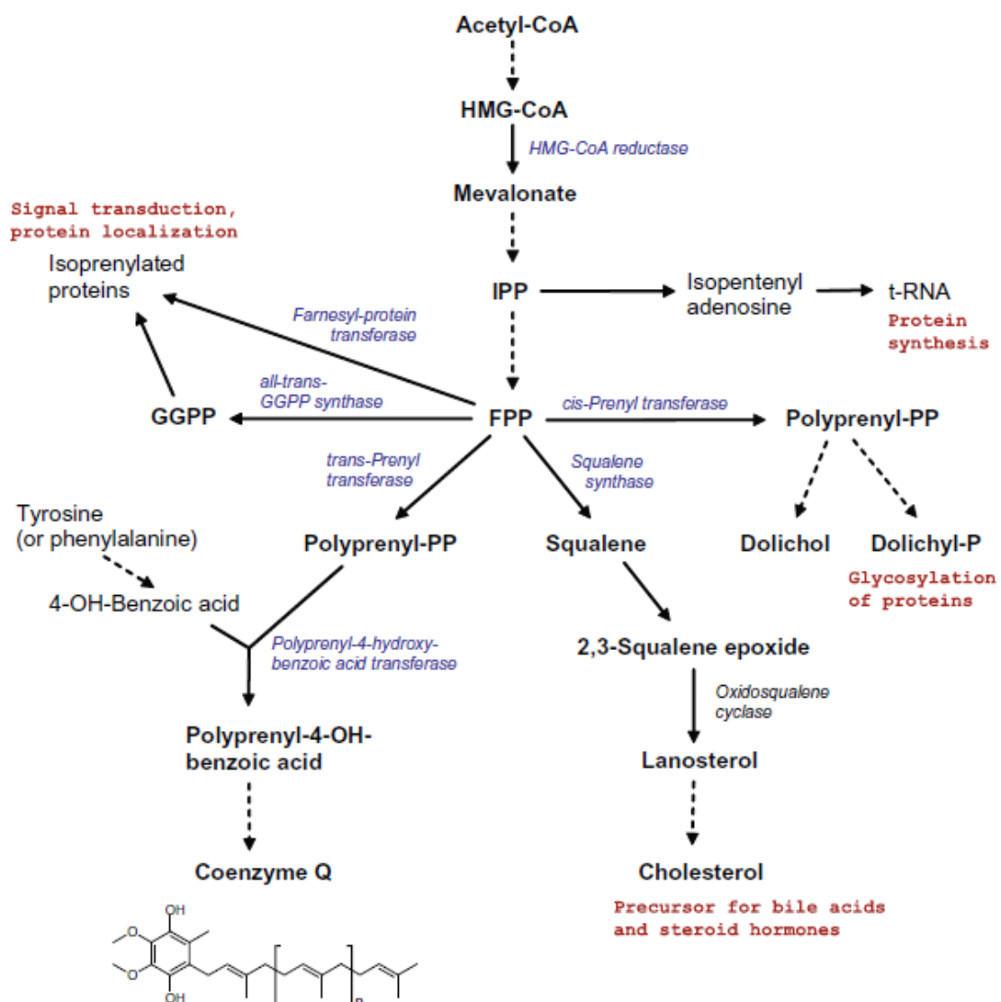
Figure 6 – La voie du mévalonate, qui aboutit à la formation de FPP, précurseur de plusieurs molécules. Les enzymes indiquées sont celles catalysant la réaction limitante. Pour le CoQ, on ne sait toujours pas laquelle des deux enzymes est limitante.
