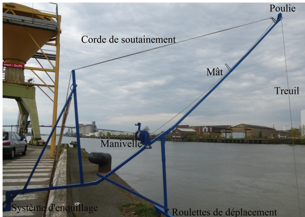
Photographie n°56 : les différents éléments d'un carret de terre – partie mât
