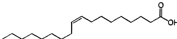
ACIDE OLEIQUE
