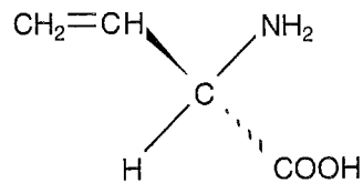
Formule de la vinylglycine
