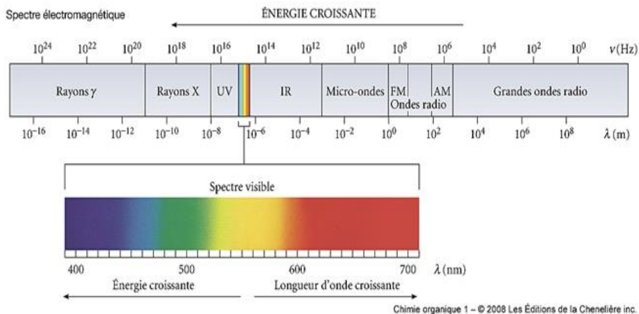
Figure 20 : Spectre électromagnétique (Site internet n°17).
