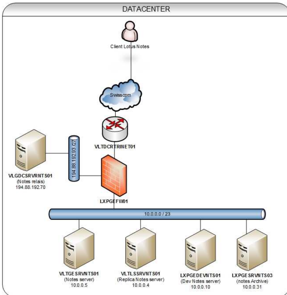
Fig. VII : Cartographie infrastructure Lotus Notes
