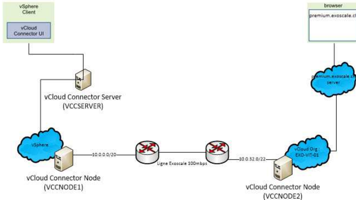
Fig XIV Synoptique Schéma réseaux (Veltigroup – Exoscale)
