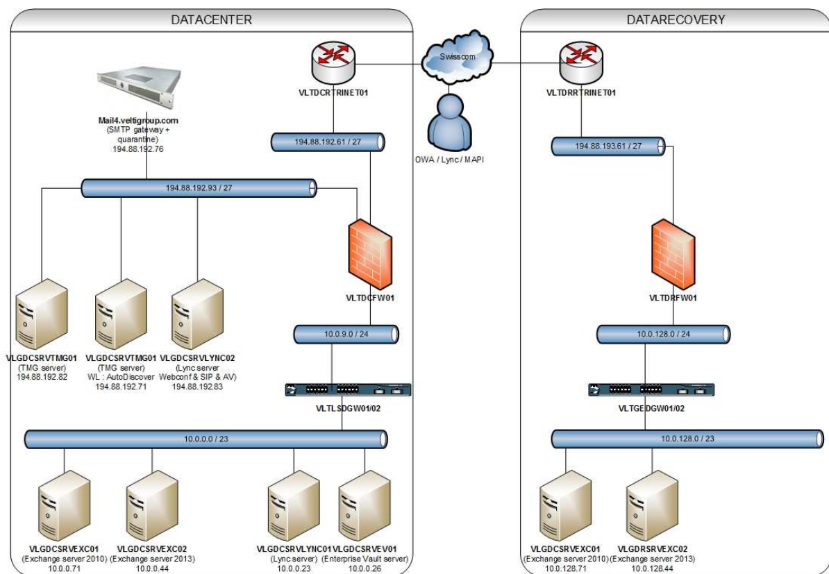
Fig. IX : Cartographie infrastructure Messagerie et Remote access
