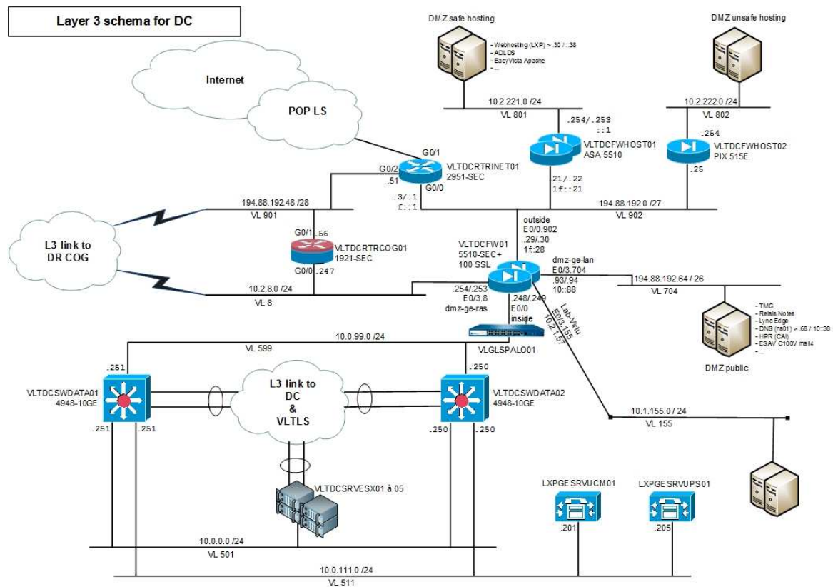
Fig. II : Schéma réseau site Datacenter
