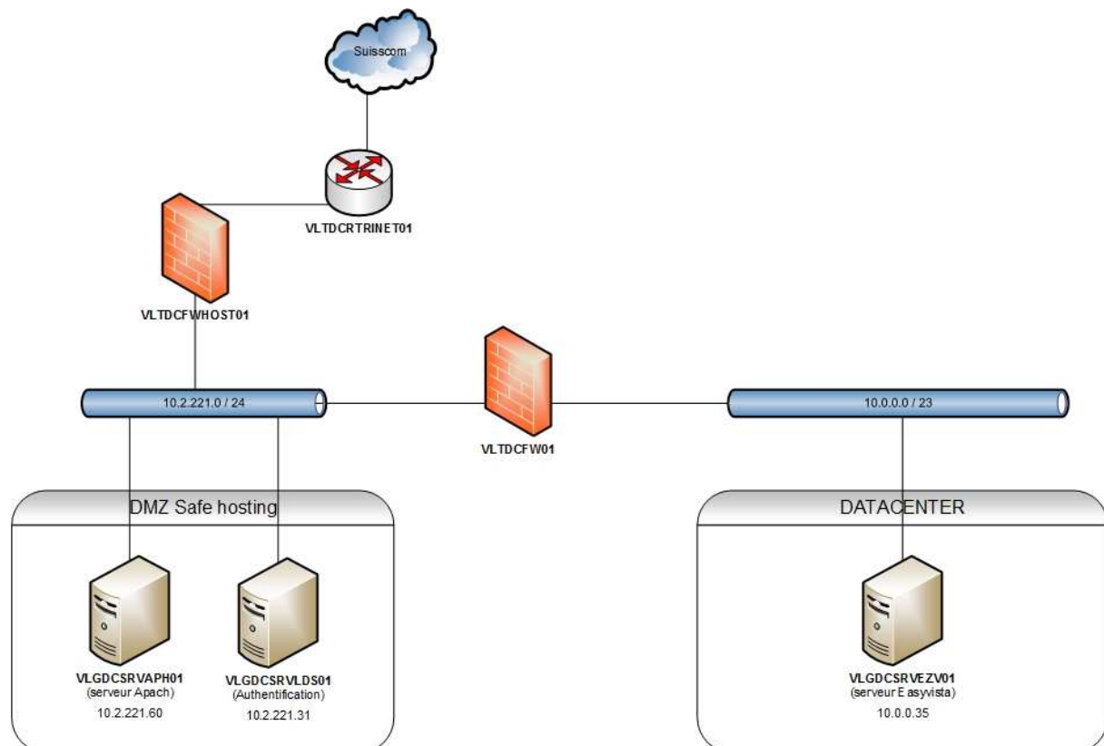
Fig. XII : Cartographie infrastructure Ticketing
