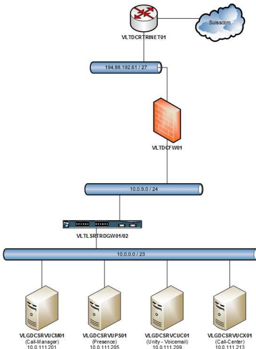
Fig. XIII : Cartographie infrastructure Téléphonie
