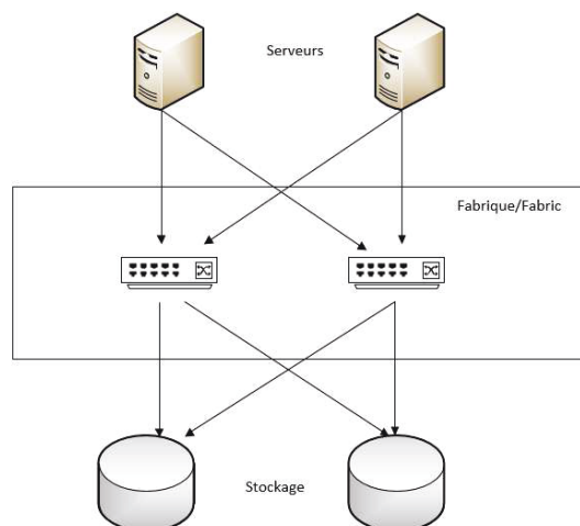
Fig. XIII : San Fabric communication
