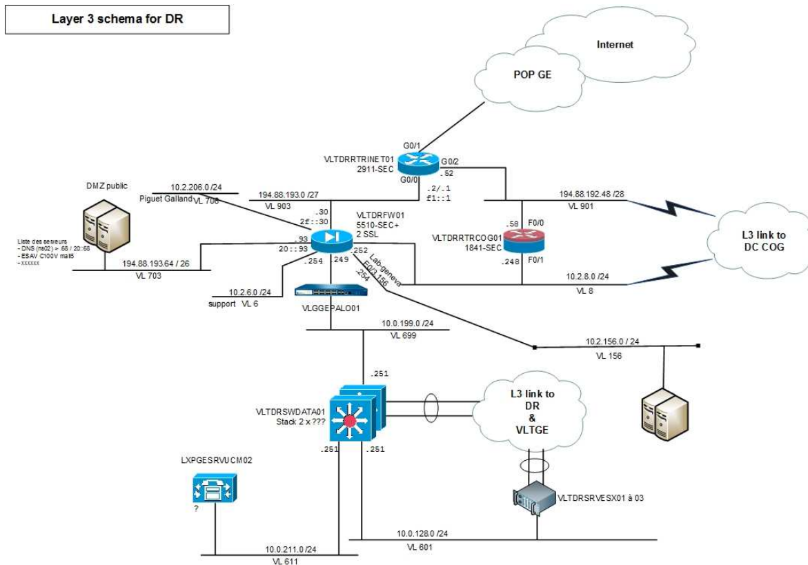
Fig. III : Schéma réseau site Datarecovery
