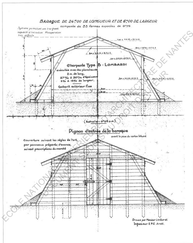
Coupe d'une Baraque préfabriquée prévue pour 60 personnes. Source René Grando, d'après « Camp d'Argeliers » op.cit.
