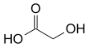
Figure 26 : Structure chimique de l'acide glycolique
