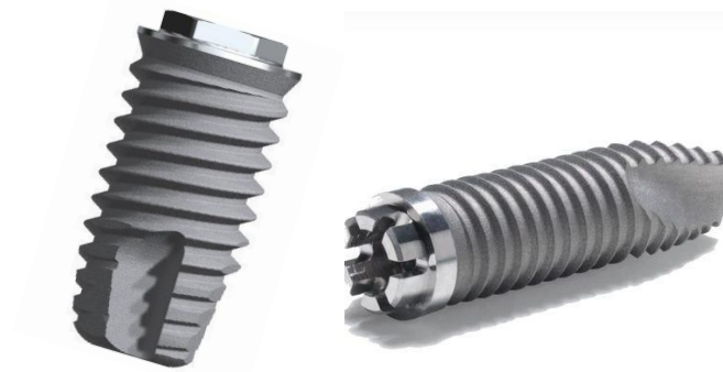
Figure 3 : implant MKIII MD à connectique externe hexagonale de Nobel Biocare à gauche ; implant SPLINE MD à connectique externe crénelée de la firme Zimmer à droite.
