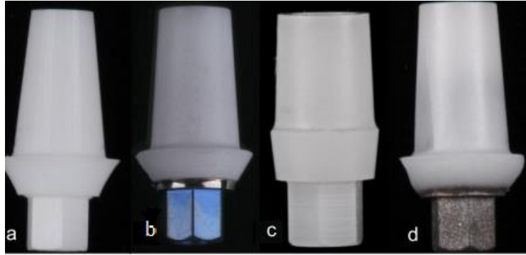
Figure 1 : (a) pilier CAD/CAM tout Zircone. (b) pilier zircone collé sur base titane. (c) pilier préfabriqué tout zircone. (d) pilier zircone solidarisé sur base titane.
