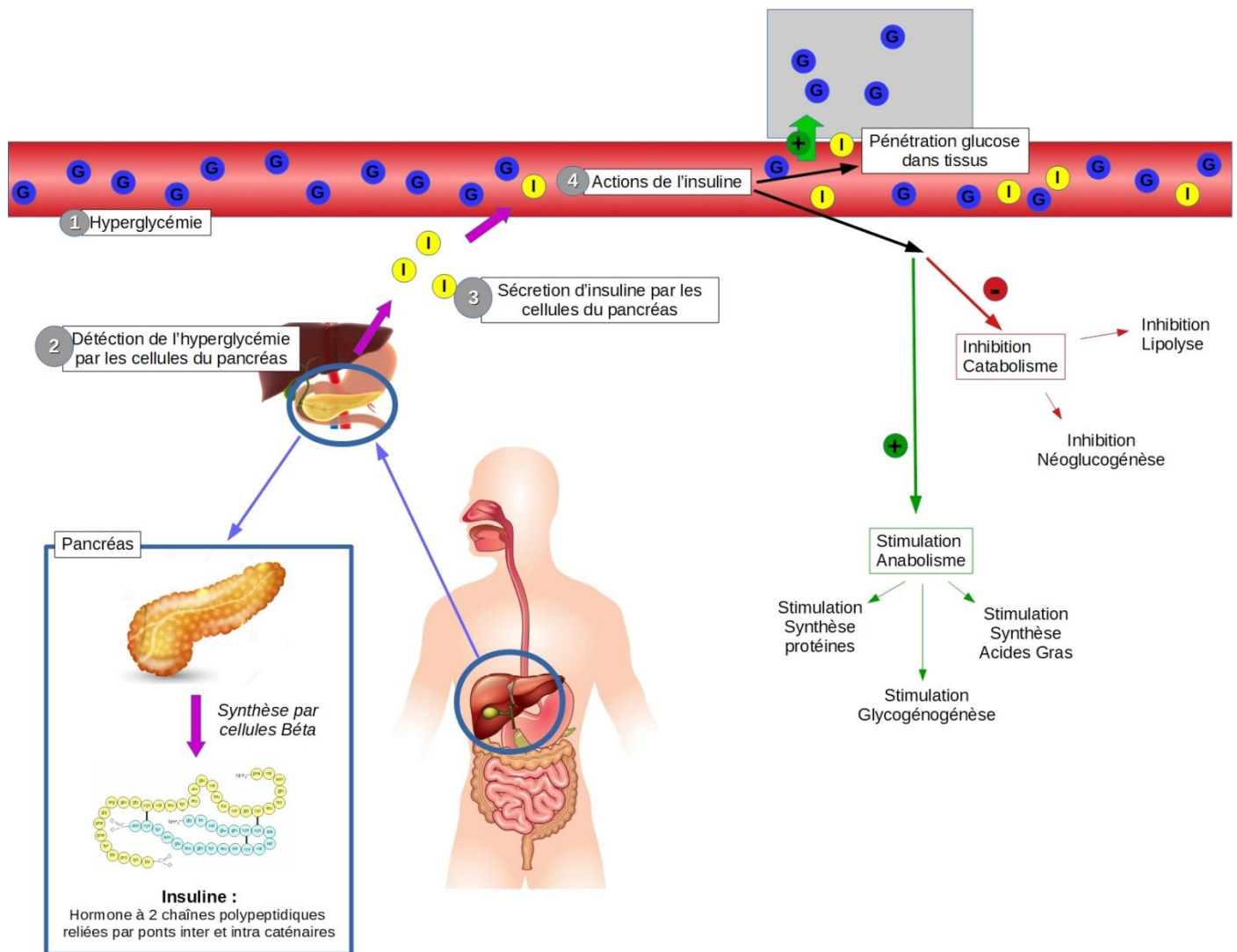
Schéma représentant le fonctionnement global de l'insuline
