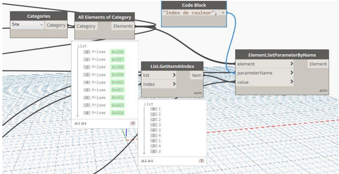
Figure 32: Script d'affectation de l'index au capteurs (Source personnelle)
