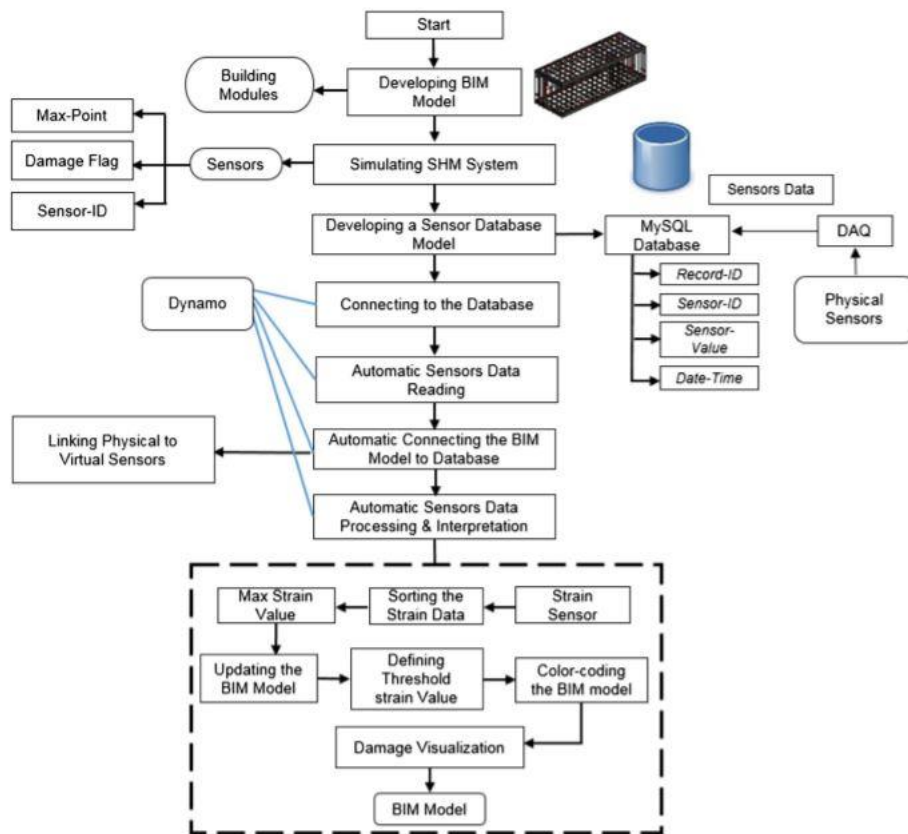
Figure 8: Hiérarchie des étapes (Source : (Valinejadshoubi al., 2019))
