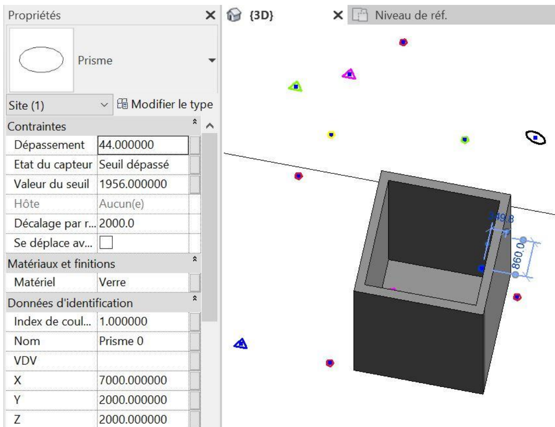
Figure 36: Résultat sur Revit (Source personnelle)
