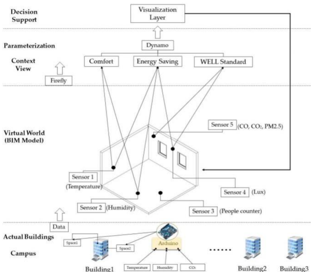
Figure 7: Etapes d'intégration des données de capteurs (Source : (Chang et al., 2018))
