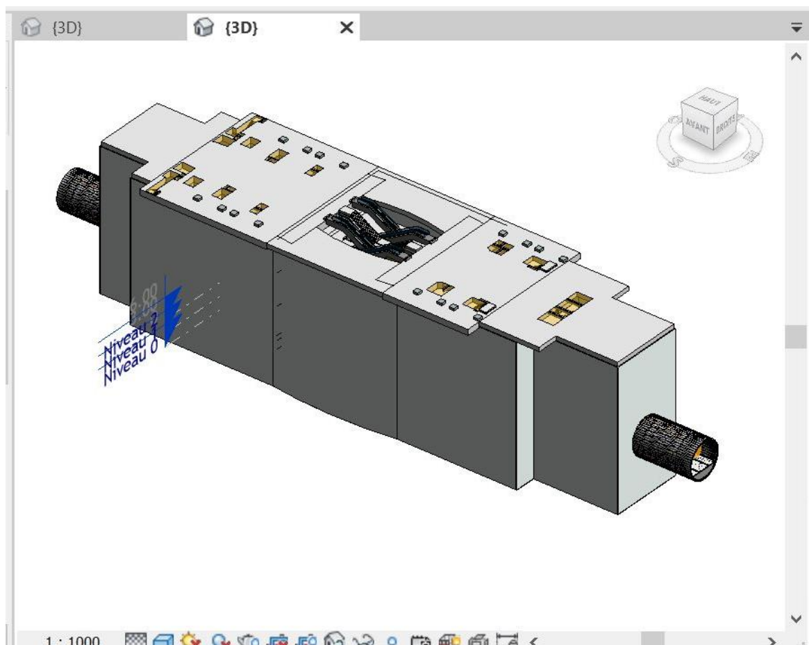
Figure 40: La maquette BIM de la gare C3C avant application du modèle ( Source: Cementys)
