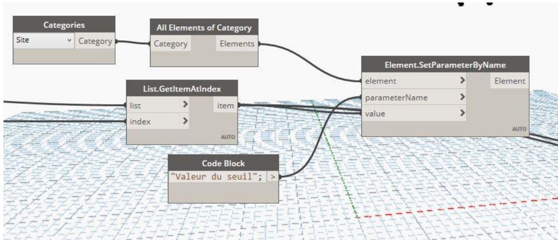
Script pour définir le paramètre «Valeur du seuil »
