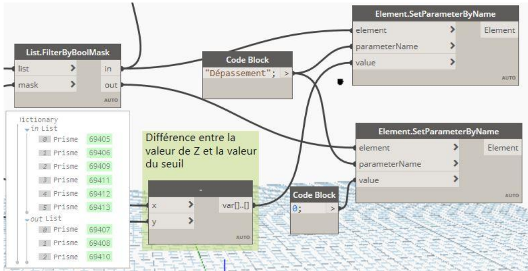
Script pour définir le paramètre « Dépassement »
