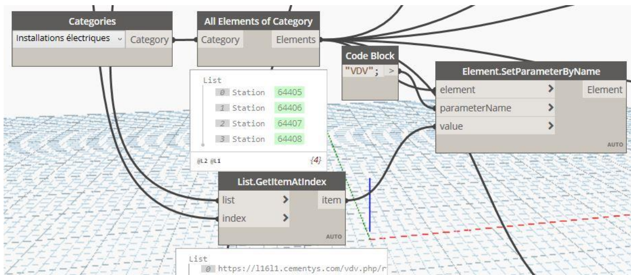
Figure 26: Script pour définir le paramètre VDV de l'élément (Source personnelle)
