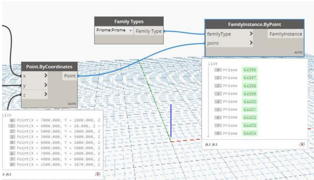
Figure 24: Script d'affectation de la famille prisme (Source personnelle)
