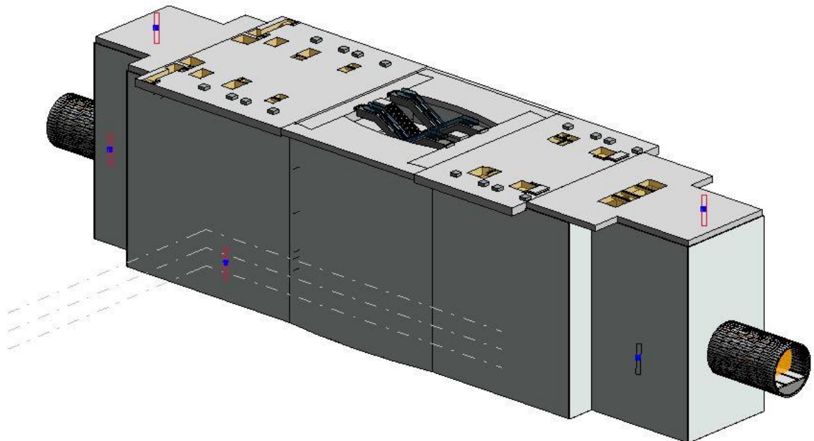
Figure 42: La maquette BIM de la gare C3C après affichage des alarmes (Source personnelle)
