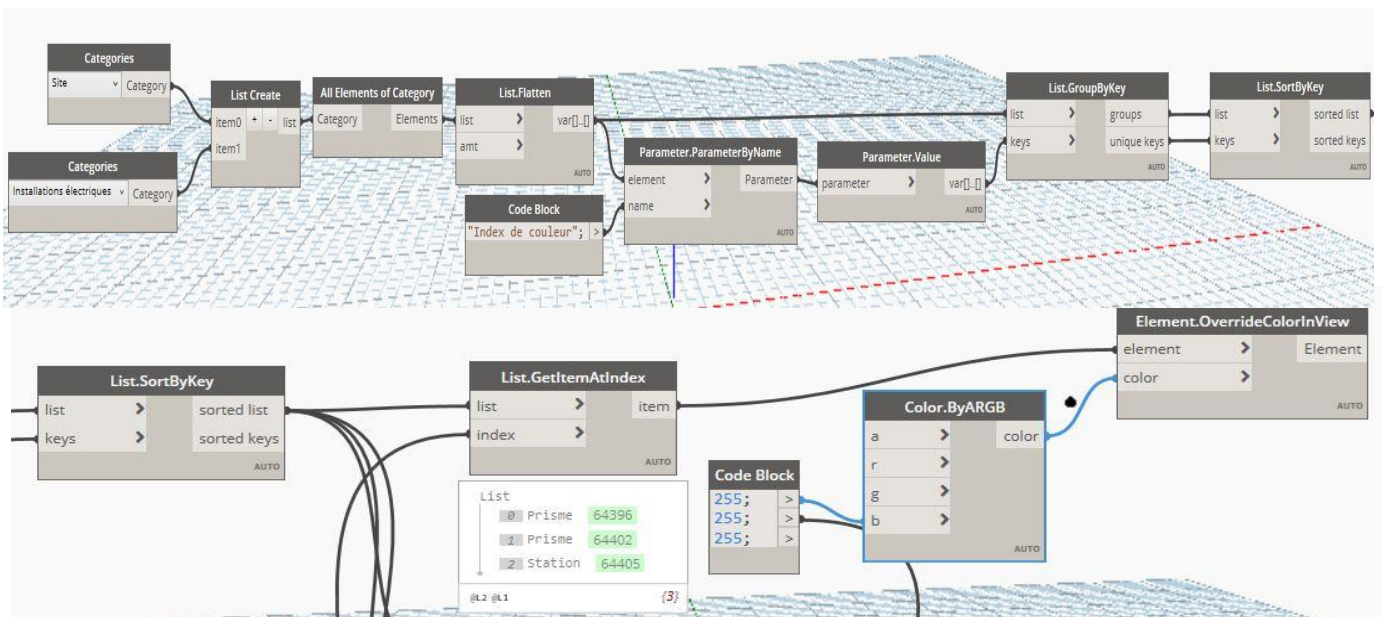
Figure 33: Script code couleur (Source personnelle)
