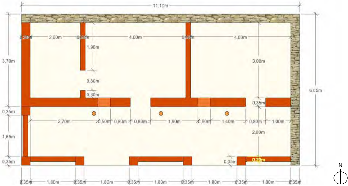
Croquis : Evaluation des coûts pour une maison témoin MCB/CRA Terre 12/12/07
