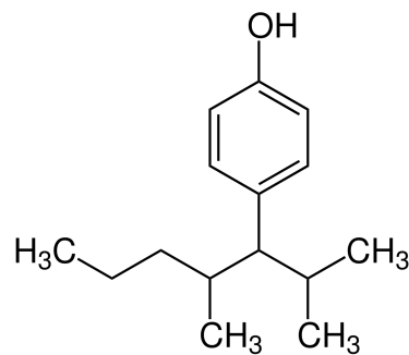
Figure 16 : Le 4-nonylphénol
