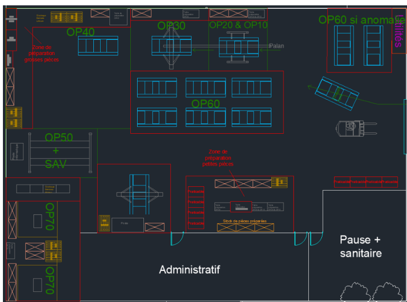
Figure 20 : Plan AutoCAD de l'hypothèse 3
