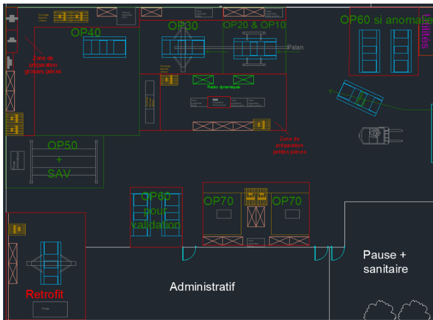
Figure 18 : Plan AutoCAD de l'hypothèse 1
