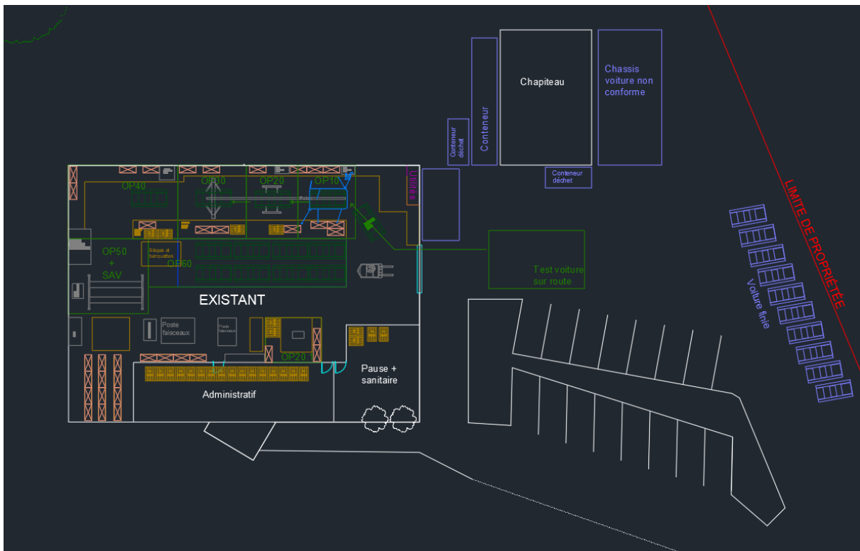
Figure 5 : Plan d'implantation mis à jour
