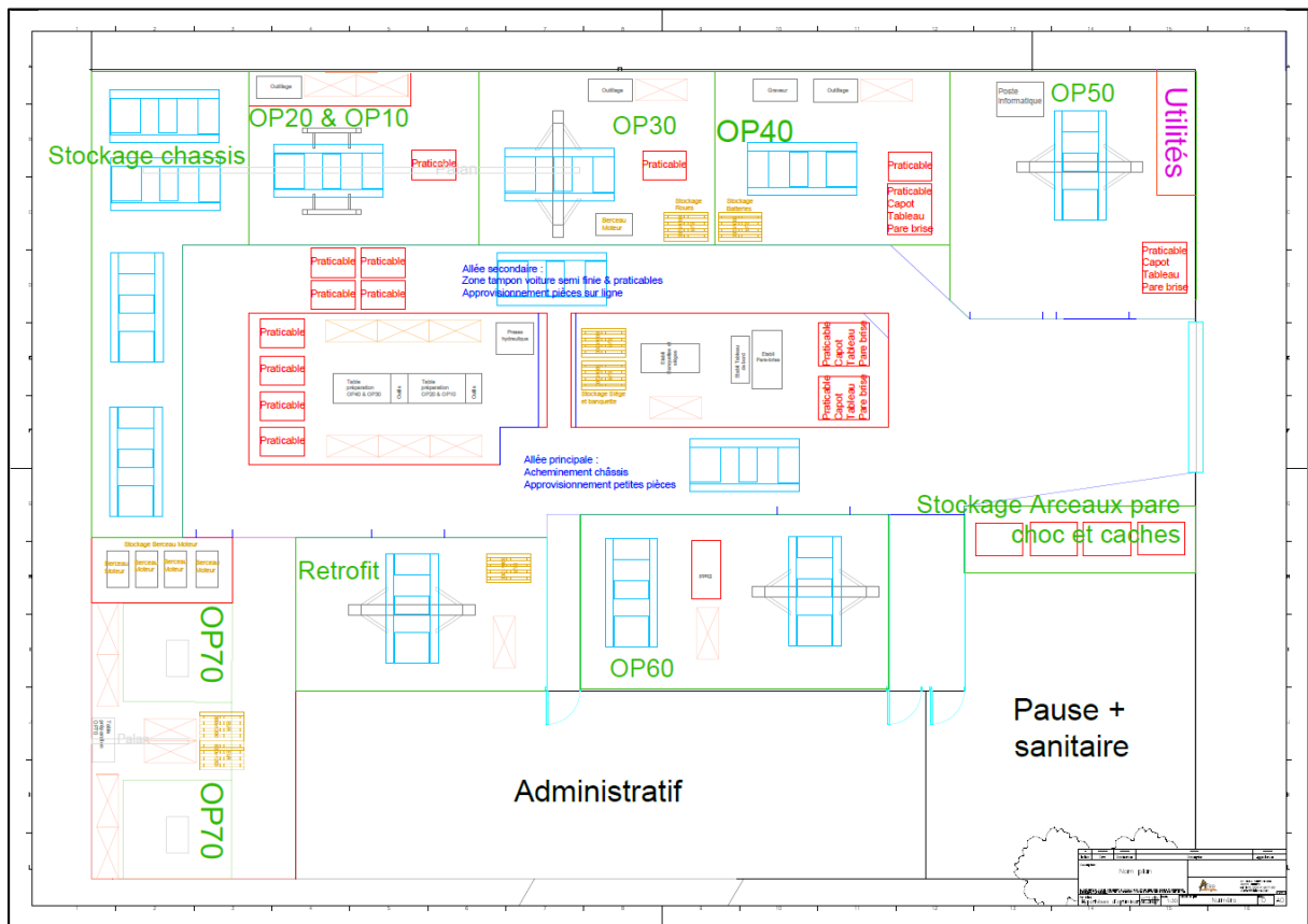
Figure 21 : Plan AutoCAD de l'hypothèse finale
