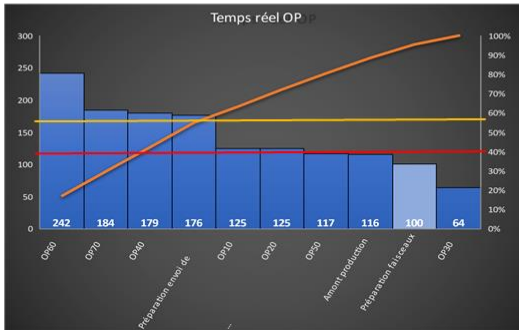
Figure 8 : Représentation graphique de Pareto du temps réel des étapes actuellement
