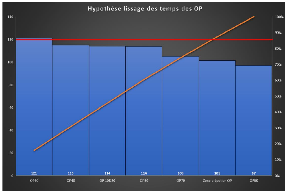
Figure 10 : Représentation graphique de Pareto du temps réel des étapes de l'hypothèse de réorganisation
