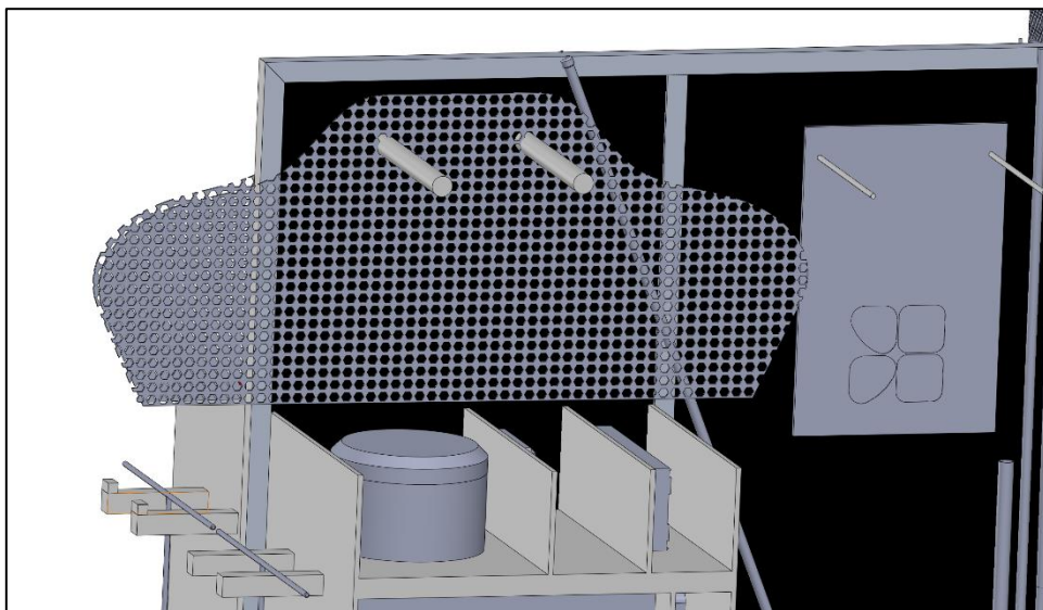
Figure 16 : Zoom sur un poka-yoké/détrompeur pour la bavette et la grille du pare choc avant
