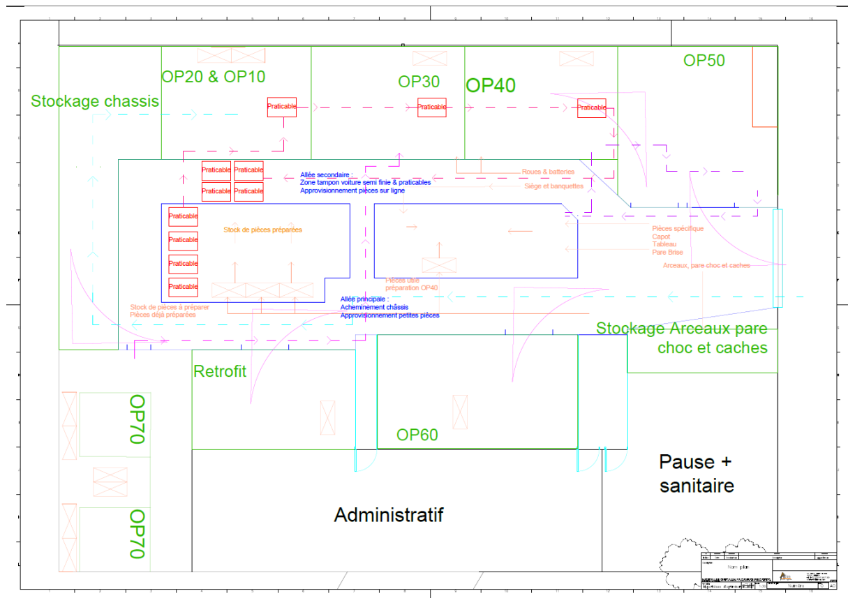
Figure 22 : Plan simplifié avec les flux de l'hypothèse finale
