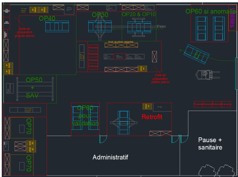
Figure 19 : Plan AutoCAD de l'hypothèse 2
