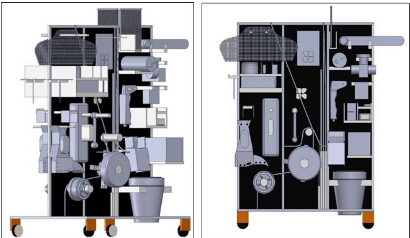
Figure 15 : Représentation 3D du chariot praticable avec toutes les petites pièces des différents OP
