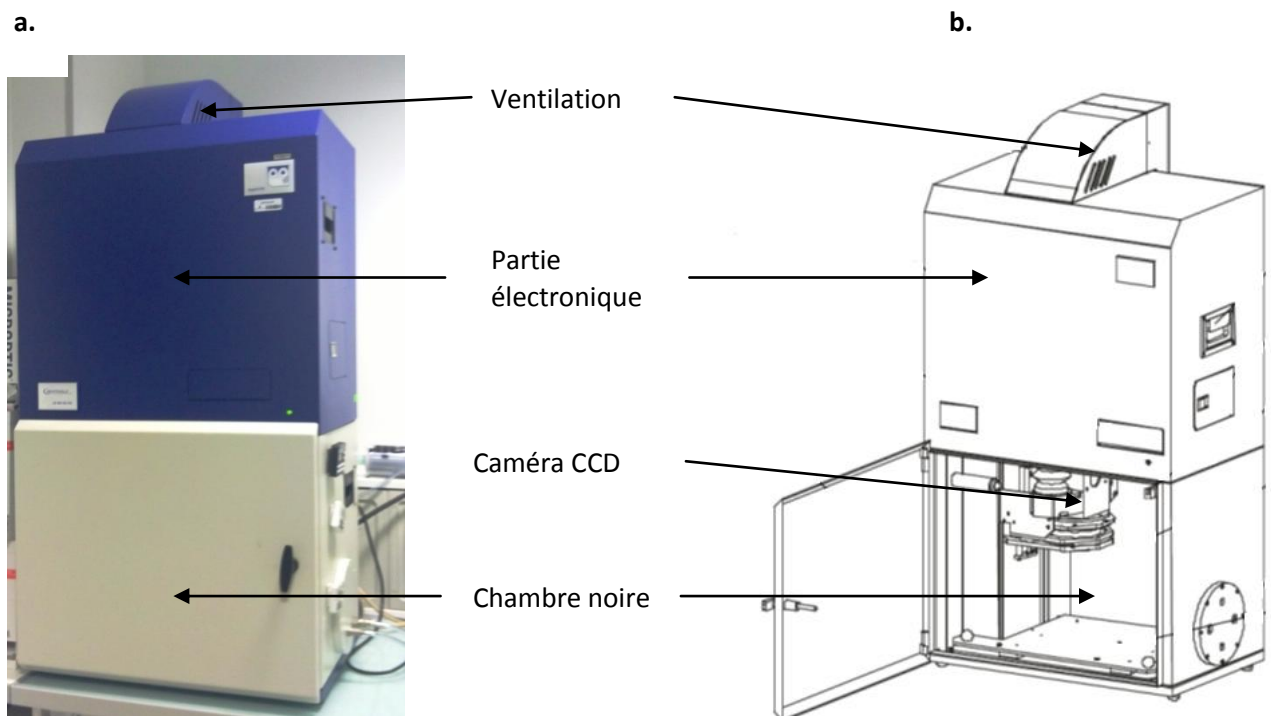
Figure 10 : Caméra CCD NightOWL II (a : cliché M. Lopez ; b: Berthold 2008)
